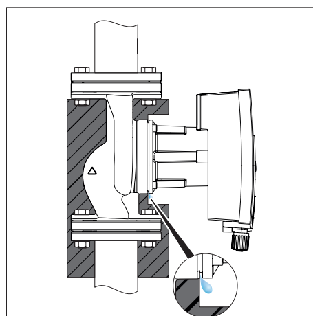
Fig. 13: Isolamento, scarico delle condense
