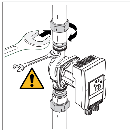
Fig. 11: Montare la pompa
