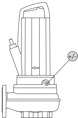
Fig. 15: Camera de etanșare: Schimb de ulei
