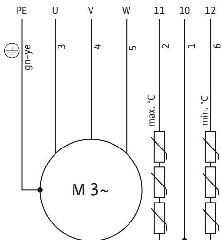
Fig. 12: Kablingsskjema: Trefasevekselstrømsmotor P17, direktestart, PTC-sensor
