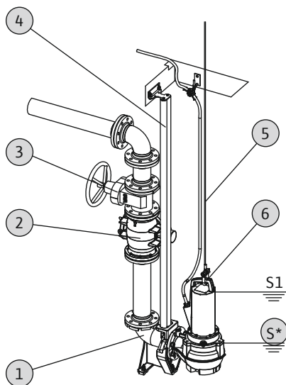
Fig. 5: Nedsenkbare installasjon, stasjonær
