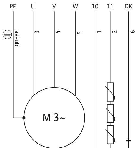
Fig. 10: Kablingsskjema: Trefasevekselstrømsmotor P13, direktestart, PTC-sensor
