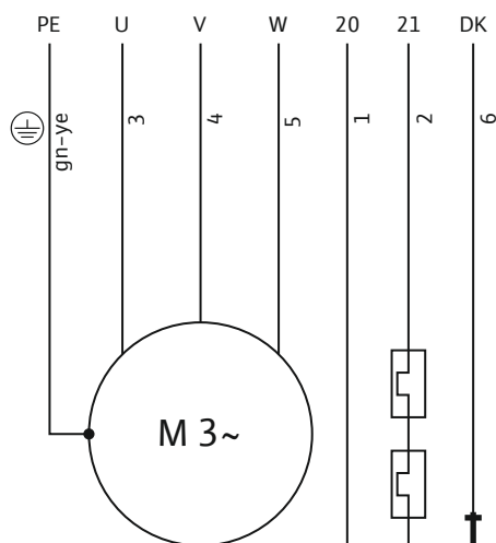
Fig. 9: Kablingsskjema: Trefasevekselstrømsmotor P13, direktestart, bimetallsensor
