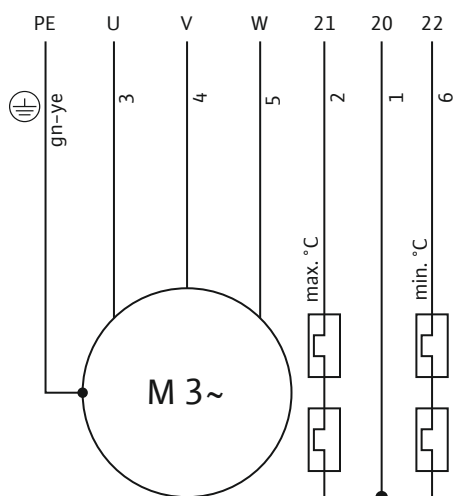
Fig. 11: Kablingsskjema: Trefasevekselstrømsmotor P17, direktestart, bimetallsensor
