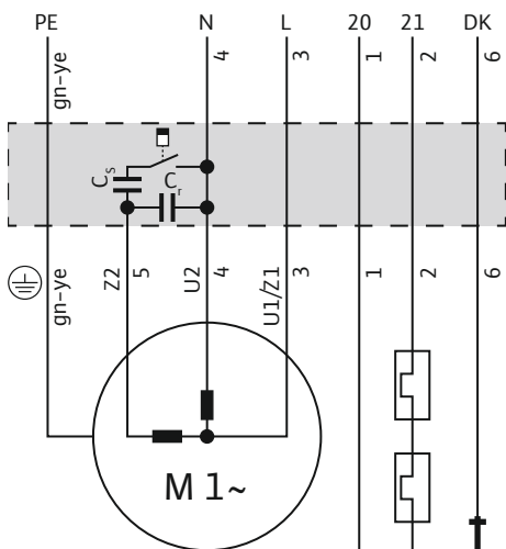
Fig. 8: Kablingsskjema vekselstrømsmotor
