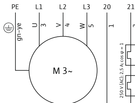
Fig. 8: Anslutningsschema trefasmotor
