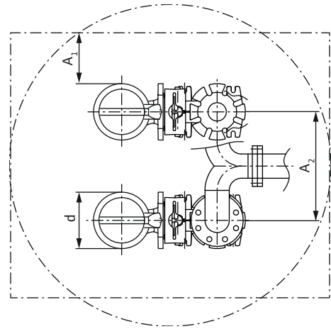
Fig. 3: Odstępy minimalne
