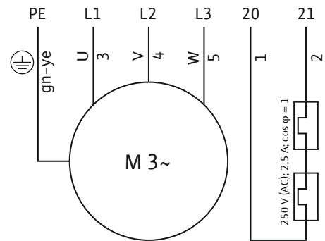
Fig. 8: Aansluitschema draaistroommotor
