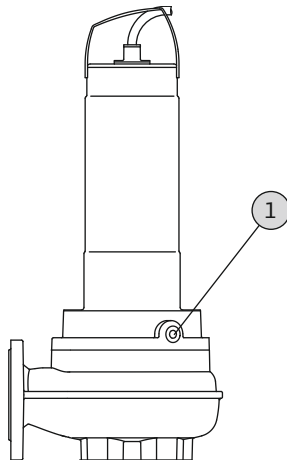
Fig. 9: Afdichtingsruimte: Olieerversen
