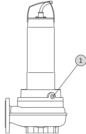
Fig. 4: Afdichtingsruimte: Olie controleren
