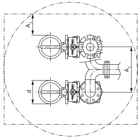
Fig. 3: Ελάχιστες αποστάσεις
