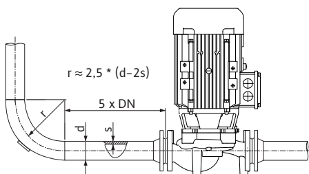
Fig. 16: Tramo de estabilización delante y detrás de la bomba
