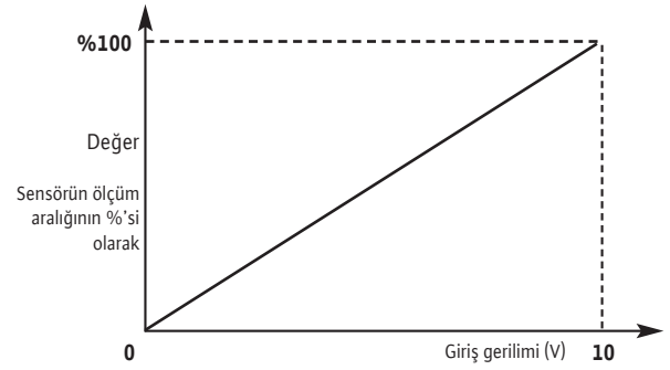
Sensör sinyali 0-10 V
