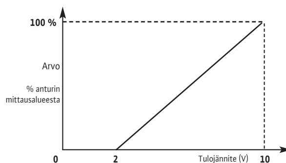
Anturisignaali 2–10 V
