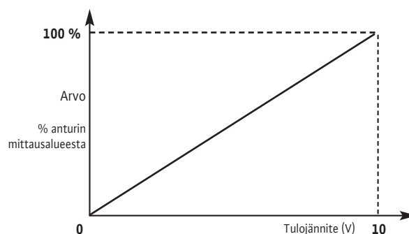
Anturisignaali 0–10 V
