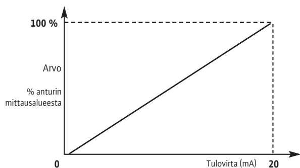
Anturisignaali 0–20 mA
