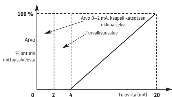
Anturisignaali 4–20 mA
