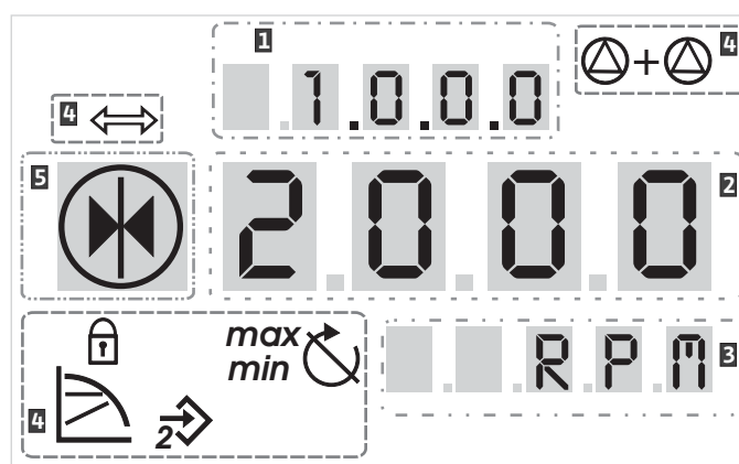
Fig. 27: Estrutura do display
