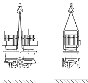
Fig. 7: Transporte da bomba
