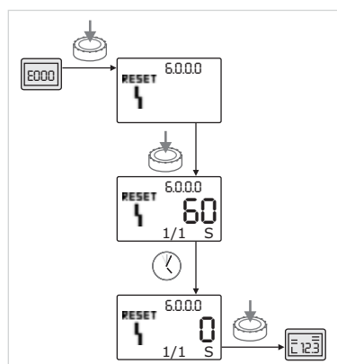
Fig. 45: Confirmar o tipo de avaria A ou D
