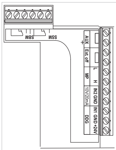
Fig. 23: Terminais de controlo
