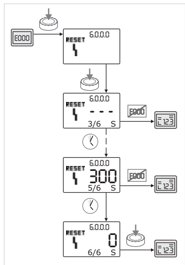
Fig. 50: Confirmar o tipo de avaria C
