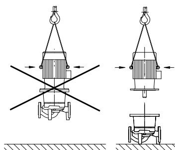
Fig. 8: Transporte do motor
