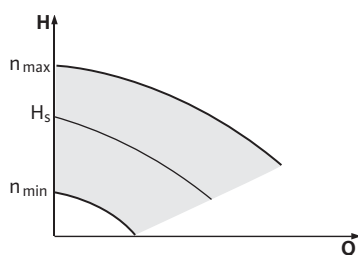
Fig. 41: Modo de controlo
