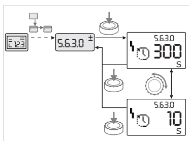
Fig. 35: Regulação com retorno ao elemento de menu “Seleccção/regulações”
