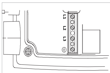
Fig. 24: Terminais de potência (terminais de ligação de rede)
