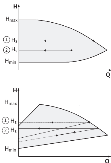
Fig. 40: Regulação \Delta p\text{-c}/\Delta p\text{-v}
