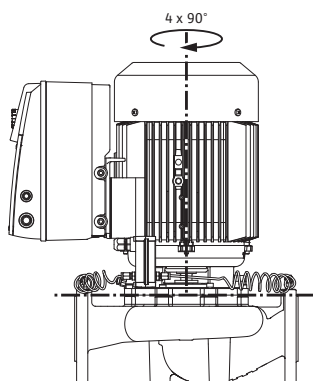
Fig. 19: Posições de instalação autorizadas com o veio do motor na vertical
