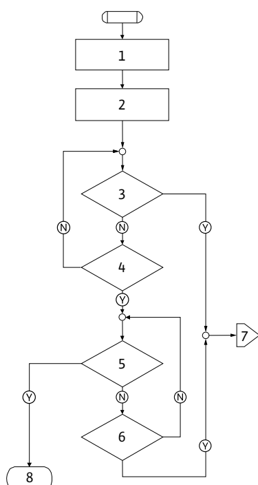
Fig. 44: Tipo de avaria D, esquema
