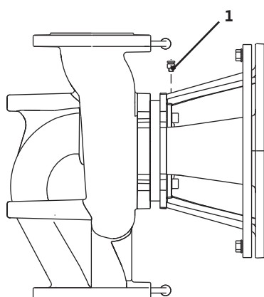
Afb. 38: Ontluchtingsventiel
