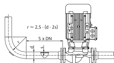
Afb. 21: Stabiliseringszone voor en achter de pomp
