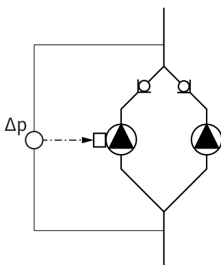
Afb. 13: Voorbeeld, aansluiting verschuldruksensor
