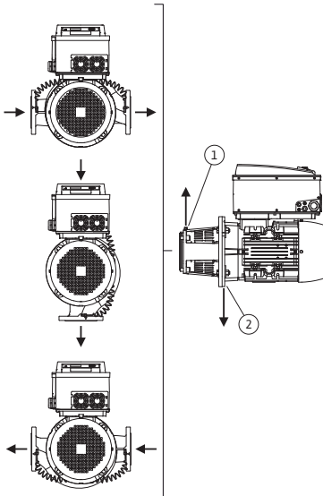
Şek. 18: Yatay motor milinde izin verilen montaj konumları
