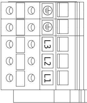
Şek. 26: Elektrik şebekesi bağlantı klemensleri (Şebeke bağlantı klemensleri)
