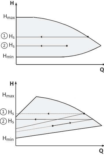
Şek. 43: Regülasyon \Delta p-c/\Delta p-v
