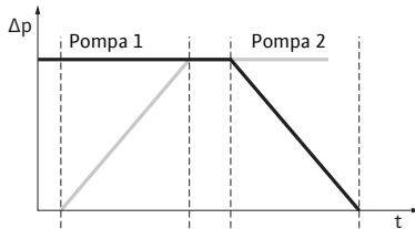
Şek. 16: Pompa değişimi
