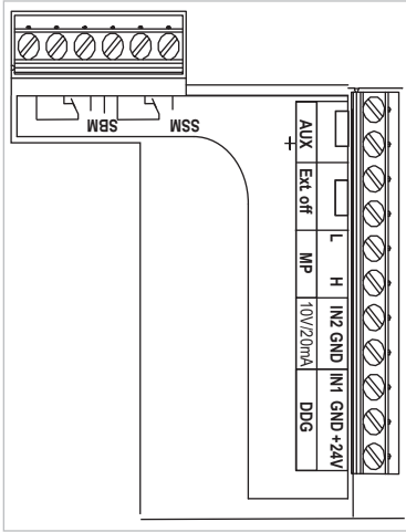
Şek. 25: Kumanda Klemensleri
