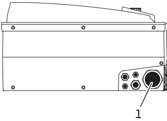
Şek. 23: Kablo bağlantısı M25/M40
