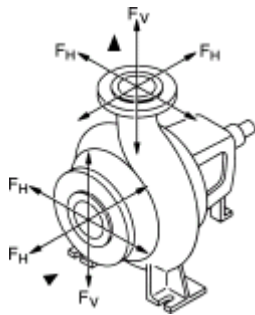
Şek. 22: Ağızlığa etki eden kuvvetler
