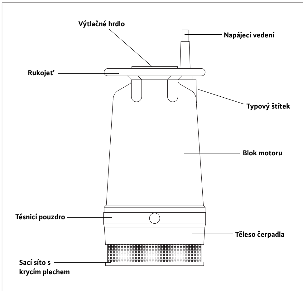
Obr. B-1: Konstrukční provedení KS37Z
