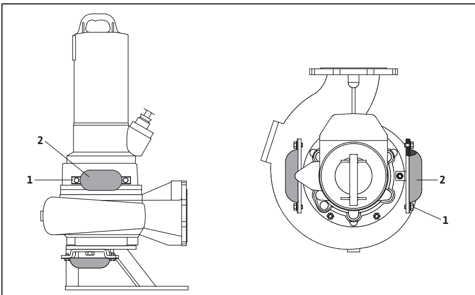
Obr. E-1: Příklady montáže obětovaných anod
