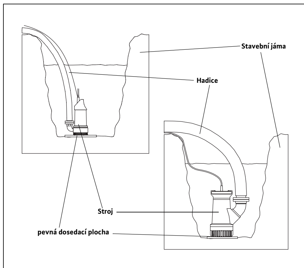
Obr. 5-1: Volná vestavba s hadicovým spojením
