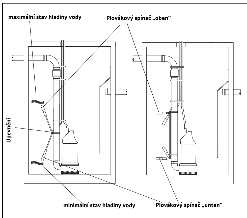
Obr. 5-4: Úroňové ovládání s jedním a dvěma plovákovým(i) spínačem (spínači)
