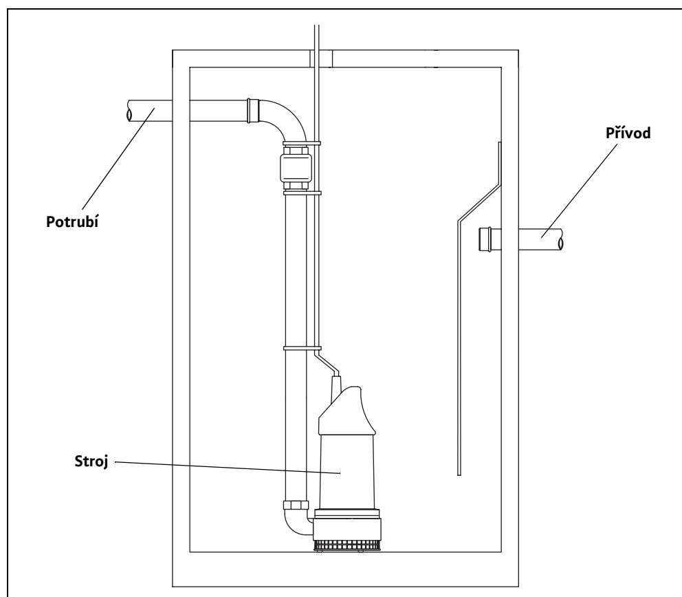
Obr. 5-3: Volná vestavba s pevným trubkovým spojením
