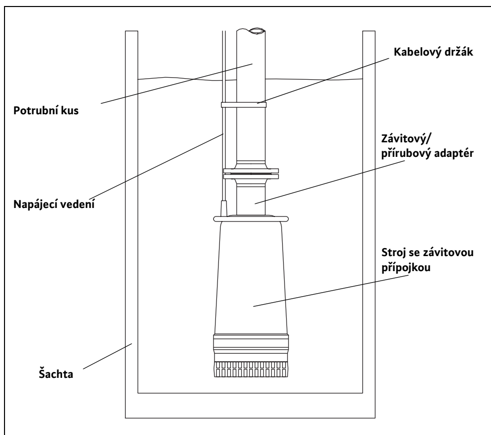
Obr. 5-2: Vestavba s volným zavěšením na potrubí – pouze s typy v provedení „Z“
