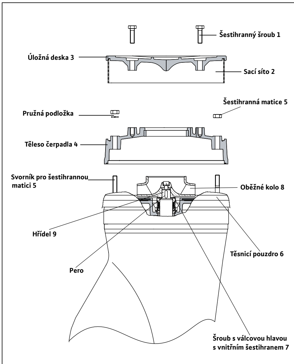
Obr. B-3: Výměna oběžného kola
