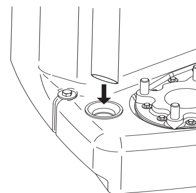
Fig. 11: Racordarea conductei de aspirație pentru pompa manuală cu membrană
