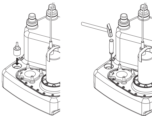
Fig. 11: Racordarea conductei de aspirație pentru pompa manuală cu membrană
