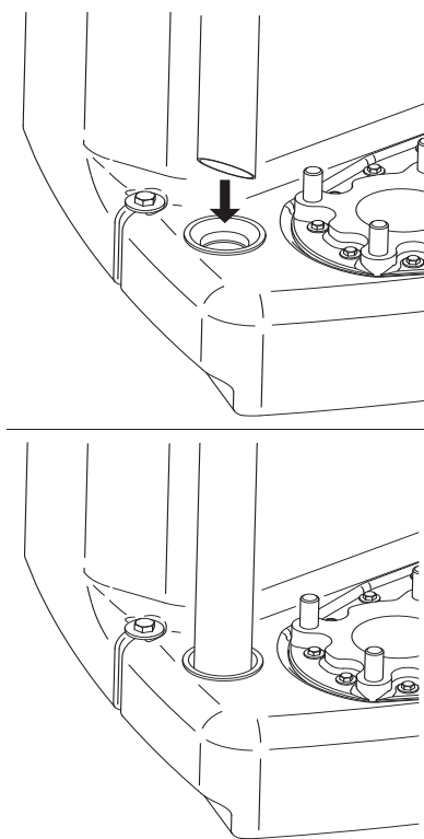
Rys. 11: Podłączenie rury ssącej do ręcznej pompy membranowej
