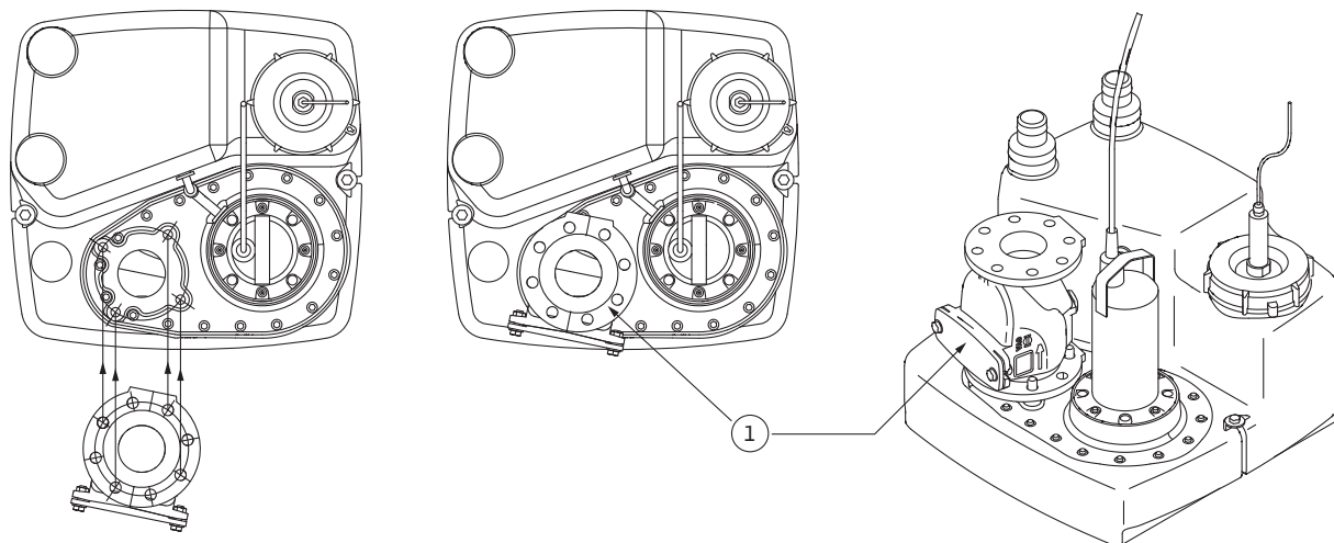
5. ábra: A visszafolyás-gátló telepítése/illesztése
