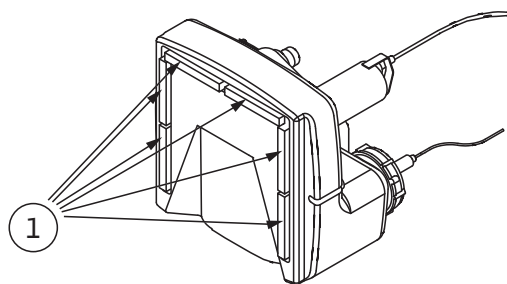
Fig. 3: Anbringung der Dämmschutzstreifen
