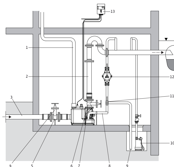
Obr. 12: Příklad instalace
