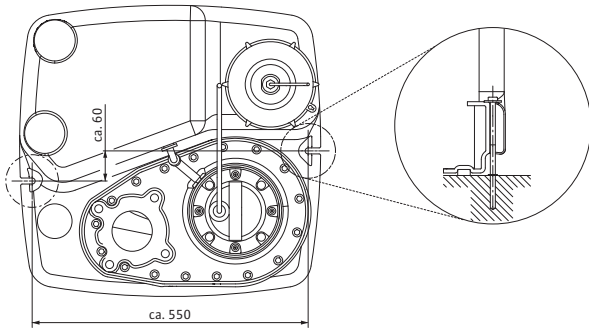
σχ. 4: Ασφάλεια έναντι άνωσης
