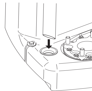
Fig. 11: Anslutning av insugningsrör för handmembranpump
