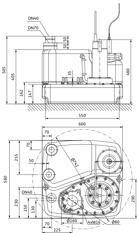
Fig. 2: Schemă de montaj
