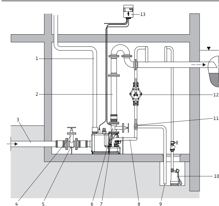
Fig. 12: Esempio installazione
