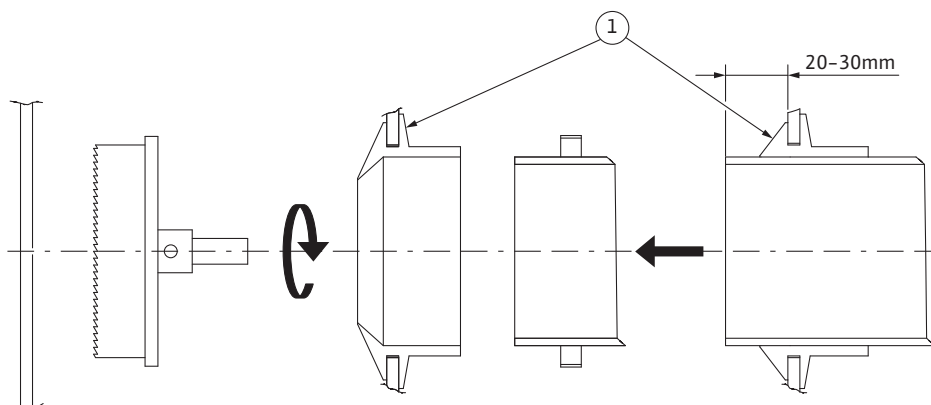
Fig. 8: Herstellung des Zulaufanschlusses DN 100 / DN 150
