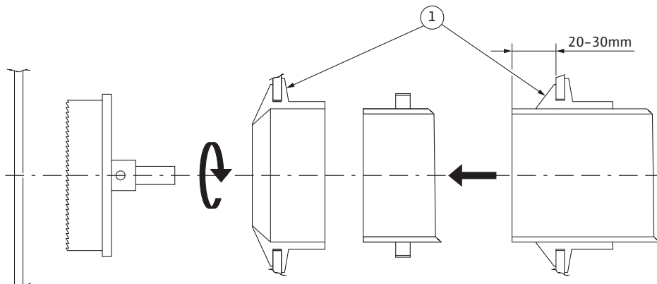
Fig. 8: Executarea racordului de admisie DN 100/DN 150
