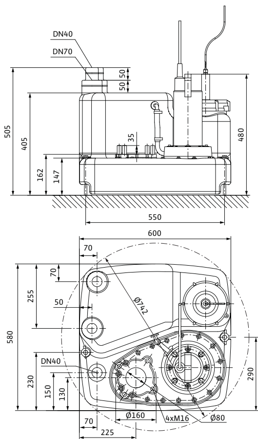
Obr. 2: Montážní výkres
