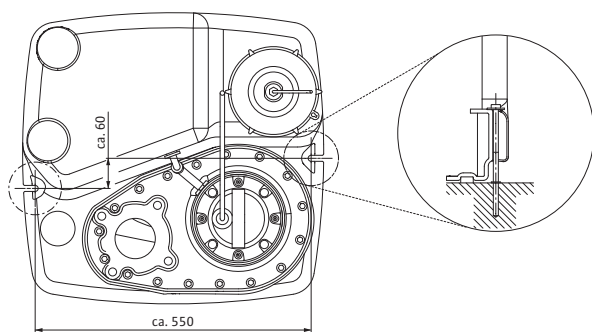
Obr. 4: Pojistka proti vztlaku
