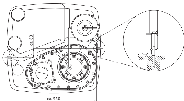
Fig. 4: Auftriebssicherung
