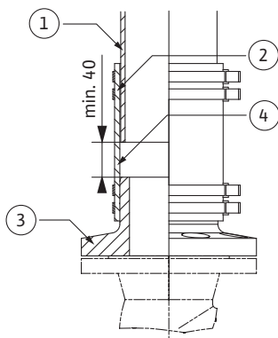
Fig. 6: Flexibler Anschluss der Druckrohrleitung
