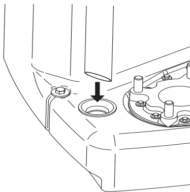
11. ábra: A kézi membránszivattyú szívócsövének csatlakoztatása
