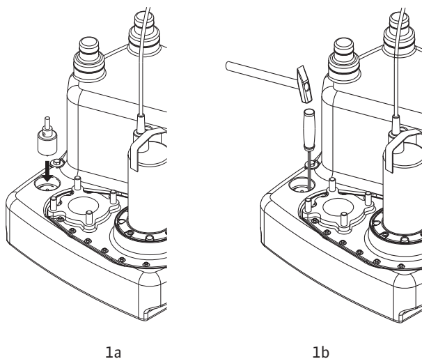
Fig. 11: Anschluss Saugrohr für Handmembranpumpe
