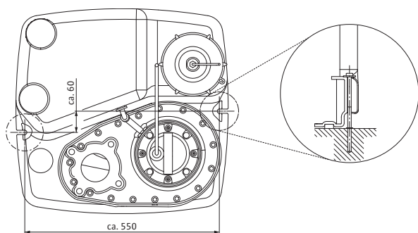
Fig. 4: Opwaartse drukbeveiliging
