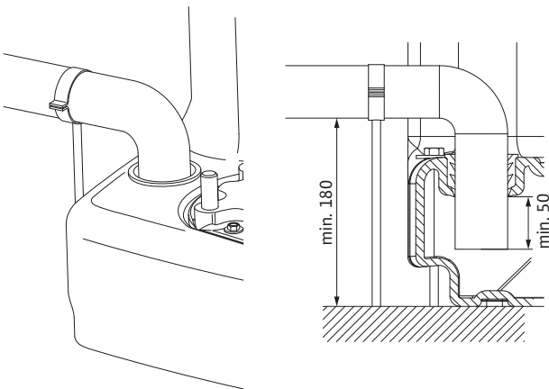
Fig. 10: Montarea conductei de admisie DN 50 la un punct de admisie inferior
