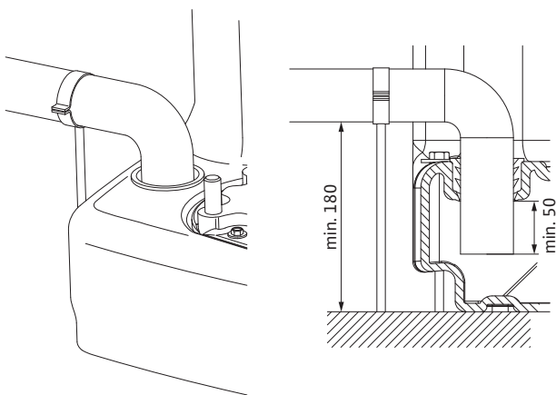
Obr. 10: Montáž nátokové trubky DN 50 k hluboké poloze nátoku
