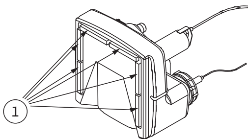
Fig. 3: Applicazione delle strisce isolanti
