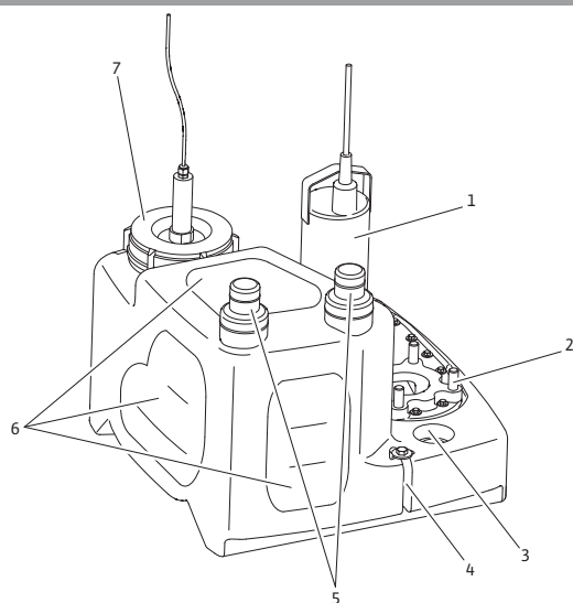
Рис. 1: Описание установки
