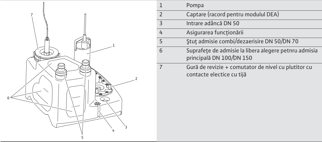
Fig. 1: Descrierea instalației
