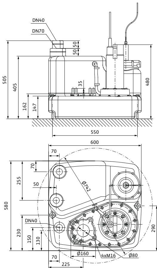
Fig. 2: Aufstellungsplan
