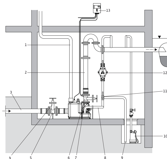
Fig. 12: Installationsbeispiel
