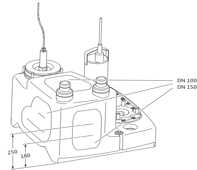
Fig. 7: Suprafețe admise pentru racordul principal de admisie DN 100/DN 150
