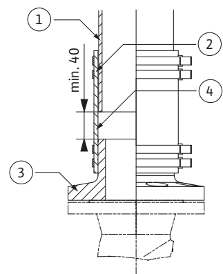
Fig. 6 : Raccordement flexible de la conduite de refoulement
