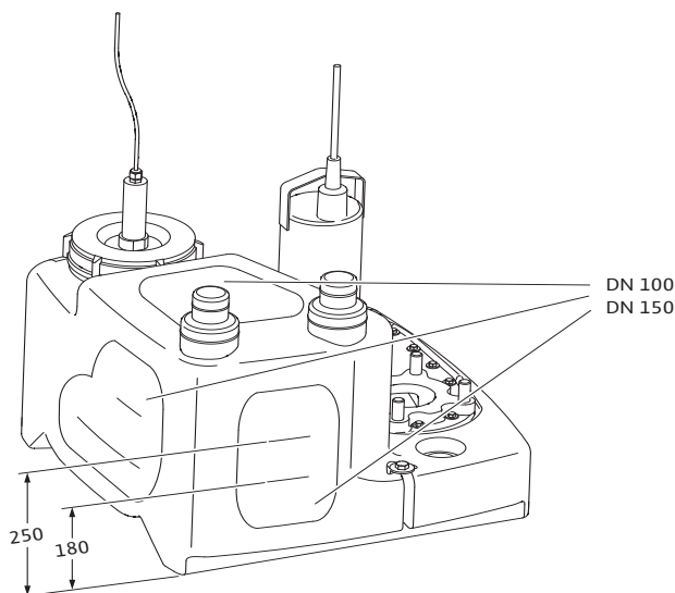
Fig. 7: Zulässige Flächen für Hauptzulaufanschluss DN 100 / DN 150
