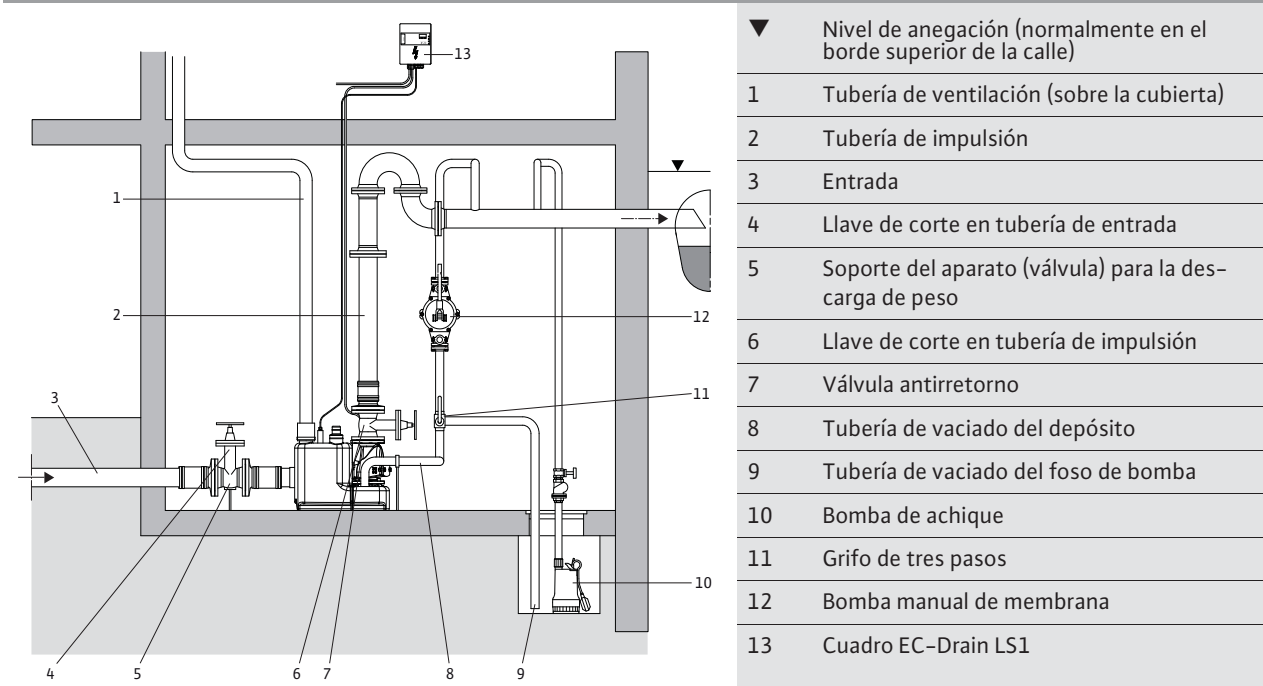
Fig. 12: Ejemplo de instalación
