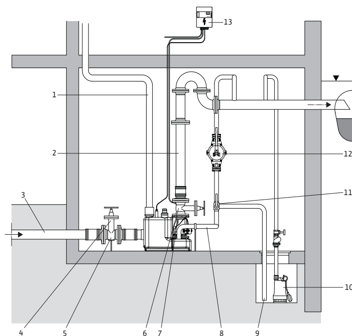
Fig. 12: Schemă de instalare
