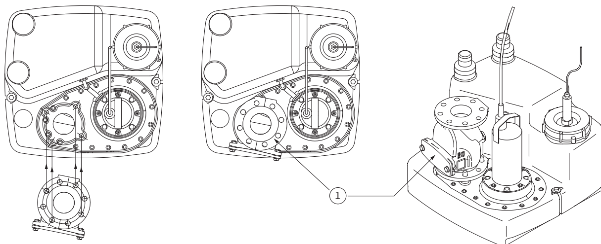
σχ. 5: Συναρμολόγηση/ευθυγράμμιση της βαλβίδας αντεπιστροφής
