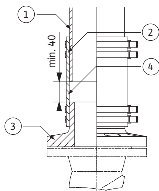
Fig. 6: Racordarea flexibilă a conduitei de refulare
