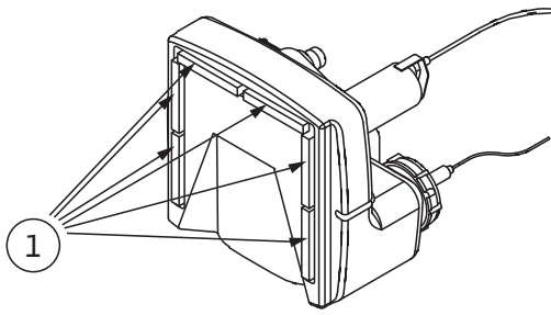
Fig. 3: Montarea benzilor de protecție izolatoare
