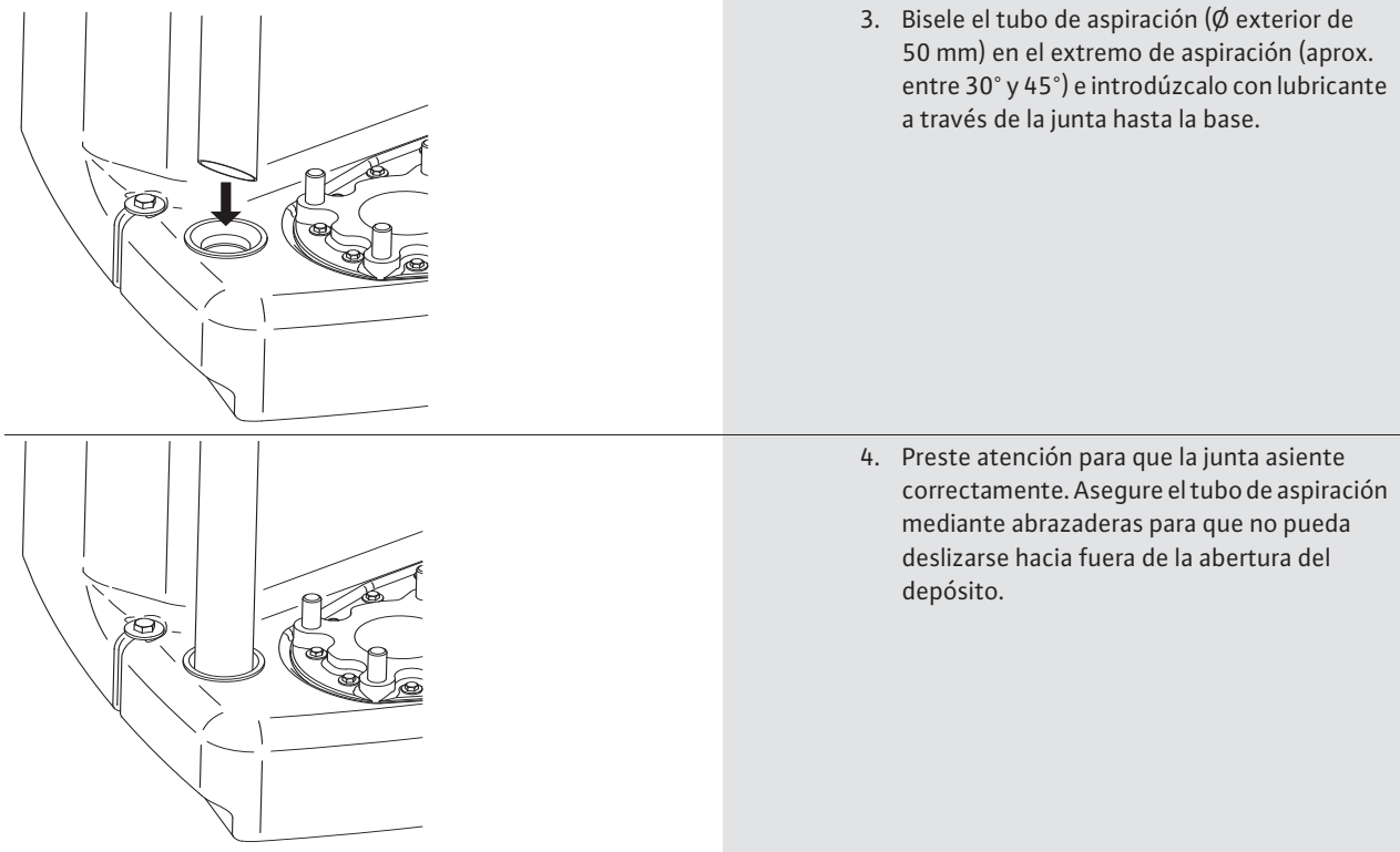
Fig. 11: Conexión del tubo de aspiración de la bomba manual de membrana
