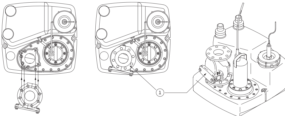
Fig. 5: Montage/Ausrichtung des Rückflussverhinderers
