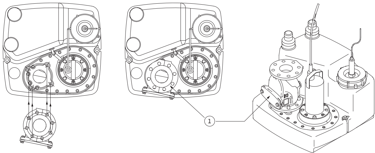
Fig. 5: Montage/orientation du clapet anti-retour
