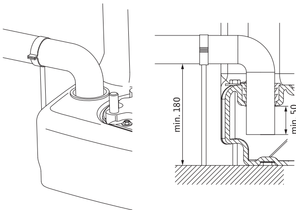
Fig. 10: Montage Zulaufrohr DN 50 an tiefer Zulaufposition
