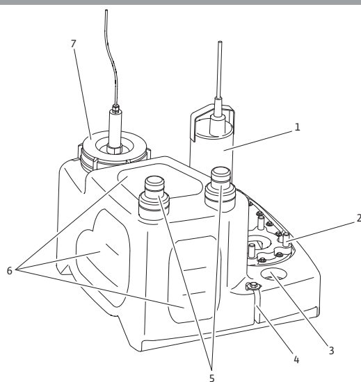
Fig. 1: Descrizione dell'impianto
