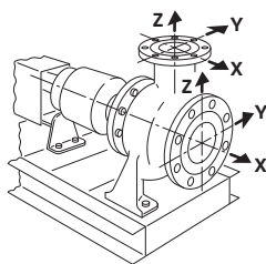
Fig. 17: 1A terhelési eset
