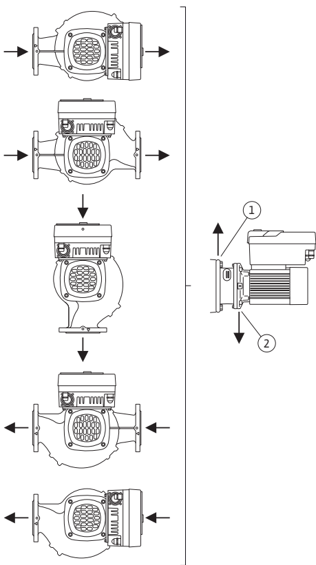
Fig. 8: Megengedett beépítési helyzetek vízszintes motortengellyel
