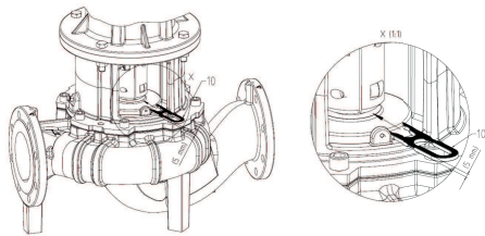
Fig. 113: A szerelő villa behelyezése
