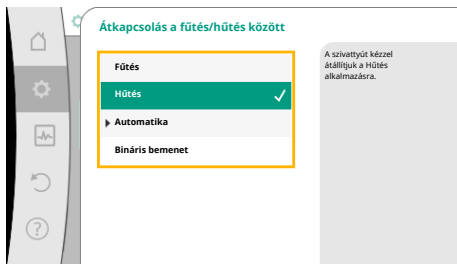
Fig. 54: Átkapcsolás a fűtés/hűtés között_Hűtés
