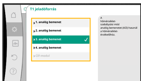
Fig. 51: A jeladó forrás hozzárendelése
