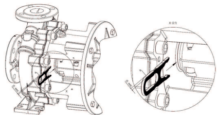
Fig. 113: A szerelő villa behelyezése
