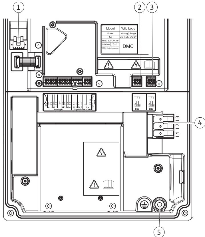
Fig. 24: A modulban található kapcsok áttekintése (11 kW – 22 kW)
