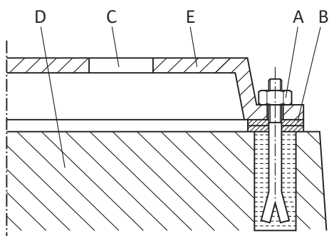
Fig. 10: Példa az alapra történő csavarozásra
