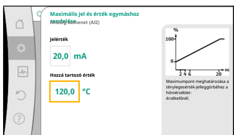
Fig. 92: Maximális jel és érték egymáshoz rendelése tényleges érték jeladó
