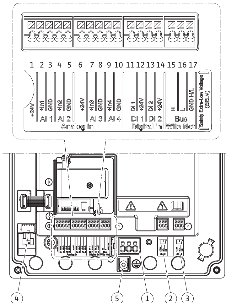
Fig. 23: A modulban található kapcsok áttekintése (0,37 kW – 7,5 kW)
