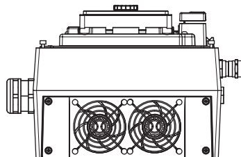
Fig. 122: Lazítsa meg a modulventilátor csavarjait.
