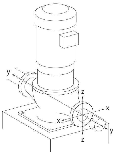
Fig. 16: 17A terhelési eset, EN ISO 5199, B melléklet
