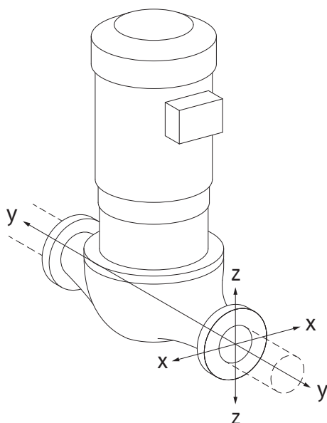
Fig. 15: 16A terhelési eset, EN ISO 5199, B melléklet
