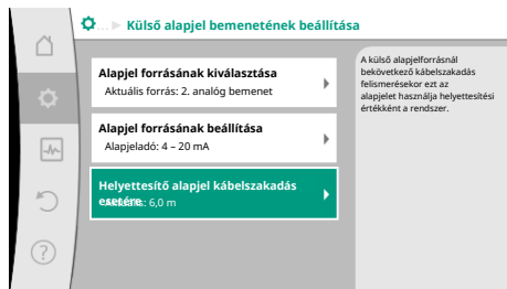
Fig. 88: Helyettesítő alapjel kábelszakadás esetére
