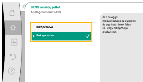
Fig. 84: Be/Ki analóg jellel
