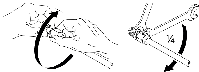
Fig. 14: A szorítógyűrű-csavarkötés 1/4-fordulattal történő továbbforgatása
