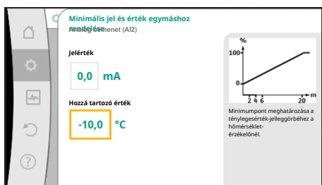
Fig. 91: Minimális jel és érték egymáshoz rendelése tényleges érték jeladó
