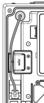
Fig. 121: A modulventilátor csatlakozókábele
