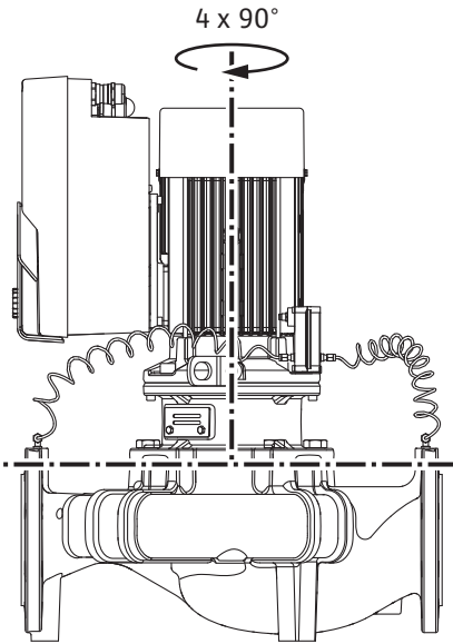
Fig. 11: Megengedett beépítési helyzetek függőleges motortengellyel
