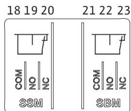
Fig. 28: Kapcsok SSM-hez és SBM-hez
