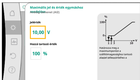
Fig. 87: Maximális jel és érték egymáshoz rendelése
