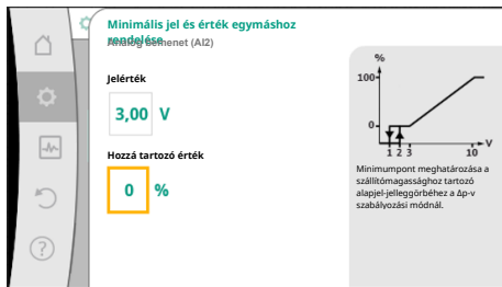
Fig. 86: Minimális jel és érték egymáshoz rendelése
