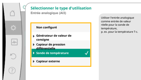
Fig. 89: Boîte de dialogue de réglage du générateur de valeur réelle
