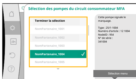
Fig. 63: Sélection des pompes secondaires pour Multi-Flow Adaptation
