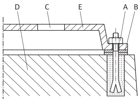
Fig. 10: Exemple de raccord fileté de fondation
