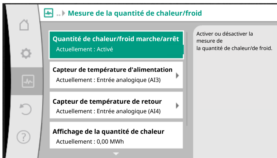
Fig. 97: Mesure de la quantité de chaleur/froid
