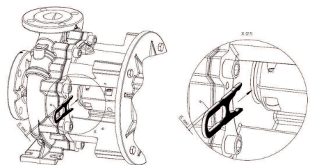
Fig. 113: Mise en place de la fourche de montage
