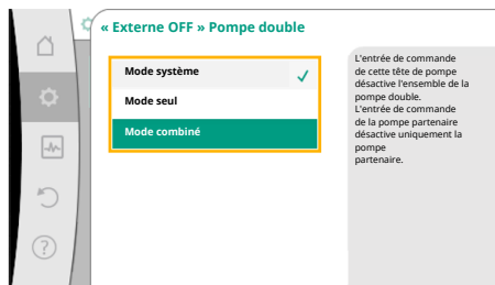
Fig. 70: Modes sélectionnables pour EXT. OFF pour les pompes doubles
