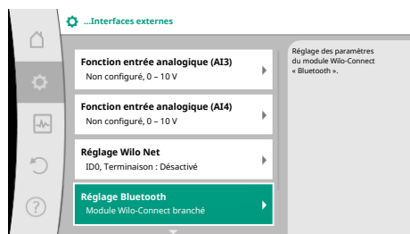
Fig. 93: Réglage de l'interface Bluetooth
