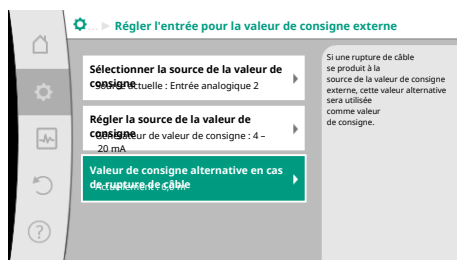
Fig. 88: Valeur de consigne alternative en cas de rupture de câble
