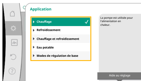
Fig. 45: Exemple de « Chauffage »
