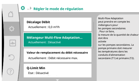
Fig. 64: Régler le mode de régulation : Mélangeur Multi-Flow Adaptation
