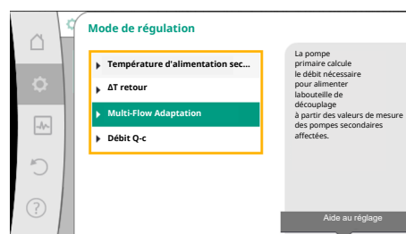
Fig. 60: Exemple : Mode de régulation « Multi-Flow Adaptation »
