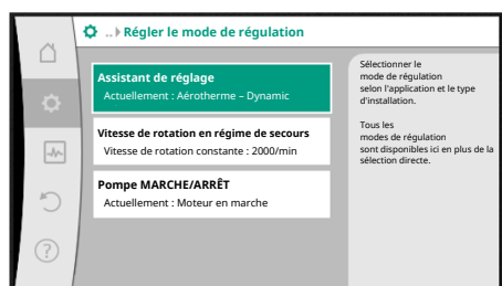
Fig. 34: Marquage vert : navigation dans le menu.
