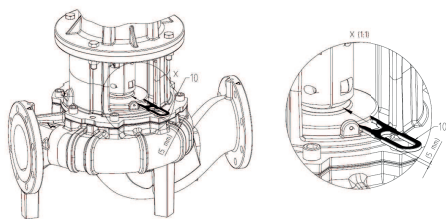
Fig. 113: Mise en place de la fourche de montage
