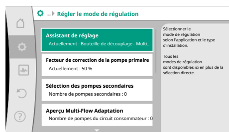
Fig. 61: Régler le mode de régulation
