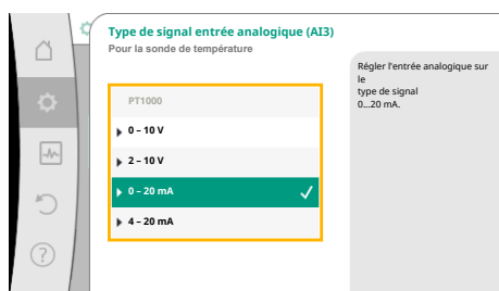
Fig. 90: Type de signal
