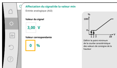
Fig. 86: Affectation du signal/de la valeur min
