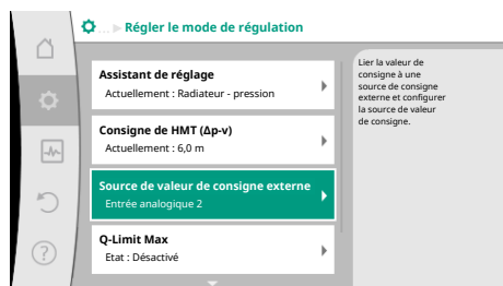
Fig. 77: Source de valeur de consigne externe
