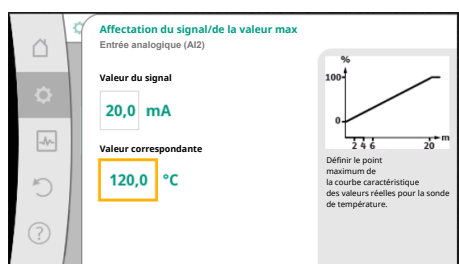
Fig. 92: Affectation du signal/de la valeur max Générateur de valeur réelle
