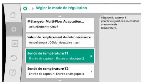
Fig. 66: Mélangeur Multi-Flow Adaptation : sonde de température
