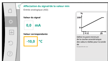
Fig. 91: Affectation du signal/de la valeur min Générateur de valeur réelle
