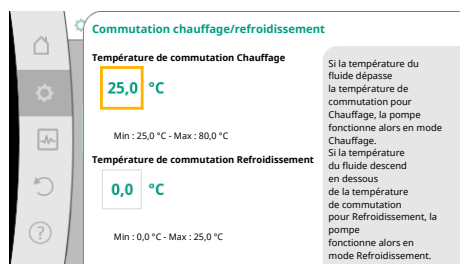
Fig. 56: Commutation Chauffage/refroidissement_Températures de commutation
