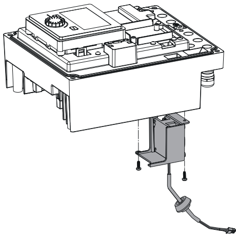
Fig. 120: Retirer le ventilateur du module, ainsi que le câble et le joint en caoutchouc
