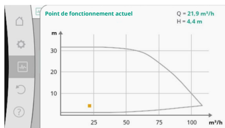
Fig. 100: Point de fonctionnement actuel
