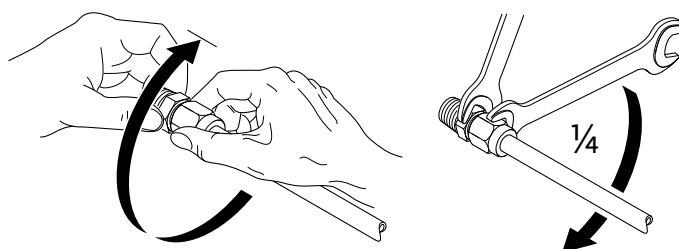
Fig. 14: Tourner la connexion par anneau de serrage d'un quart de tour supplémentaire
