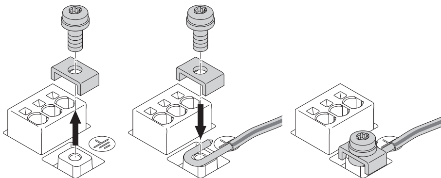
Fig. 27: Câble de raccordement rigide
