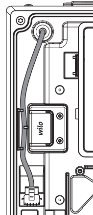
Fig. 121: Câble de raccordement du ventilateur du module
