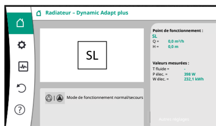
Fig. 69: Page d'accueil de la pompe double partenaire sans capteur de pression différentielle monté
