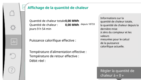
Fig. 98: Affichage de la quantité de chaleur
