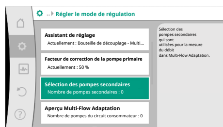
Fig. 62: Assistant de réglage – Sélection des pompes secondaires
