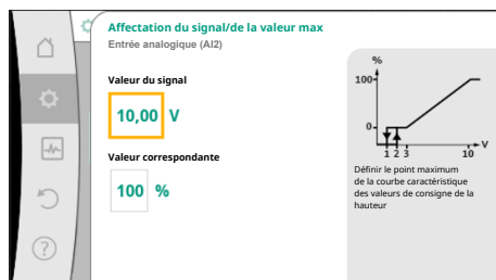
Fig. 87: Affectation du signal/de la valeur max
