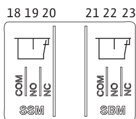
Fig. 28: Bornes pour SSM et SBM
