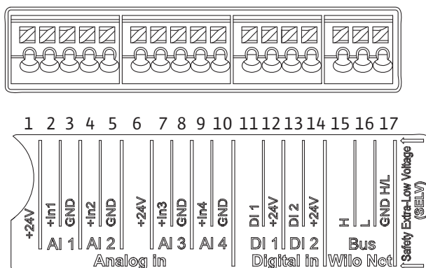
Fig. 25: Bornes pour les entrées analogiques, les entrées numériques et Wilo Net
