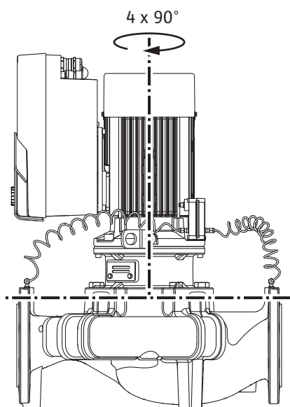
Fig. 11: Positions de montage autorisées avec arbre de moteur vertical
