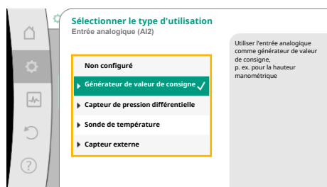
Fig. 79: Boîte de dialogue de réglage
