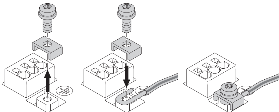
Fig. 27: Pevný přívodní kabel
