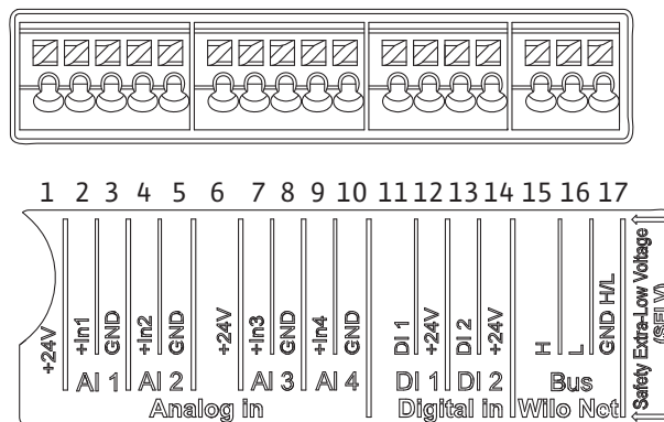
Fig. 25: Svorky pro analogové vstupy, digitální vstupy a Wilo Net
