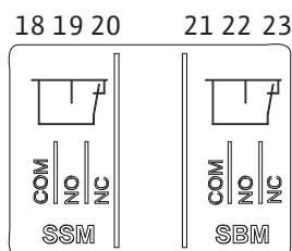
Fig. 28: Svorky pro SSM a SBM
