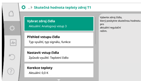
Fig. 67: Skutečná hodnota teploty zdroj T1
