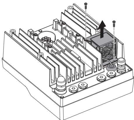
Fig. 119: Demontáž ventilátoru modulu
