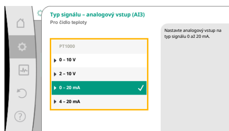
Fig. 90: Typ signálu
