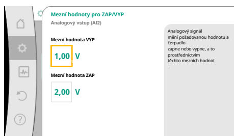
Fig. 85: Mezní hodnoty pro řízení zap/vyp prostřednictvím analogových signálů
