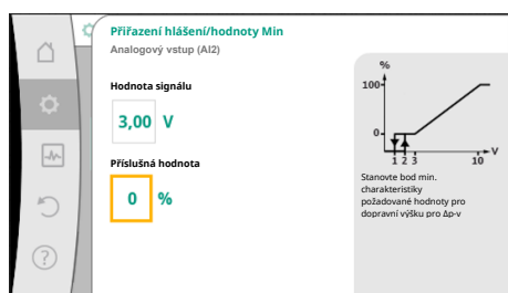
Fig. 86: Přiřazení hlášení/hodnoty Min
