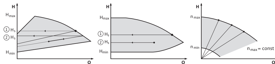
Fig. 4.2: Regulační funkce
