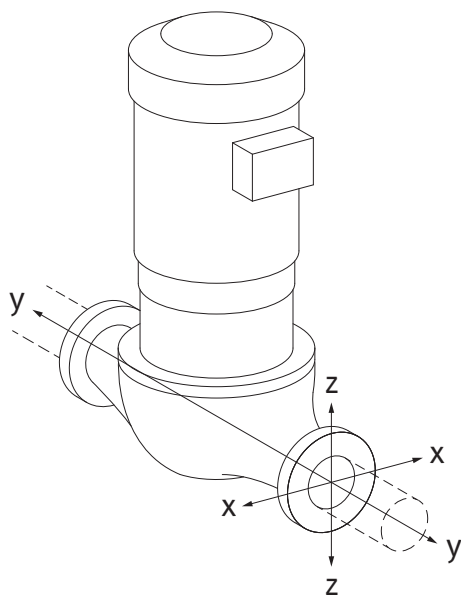
Fig. 15: Příklad zatížení 16A, EN ISO 5199, příloha B
