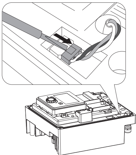
Fig. 118: Uvolnit přívodní kabel ventilátoru modulu
