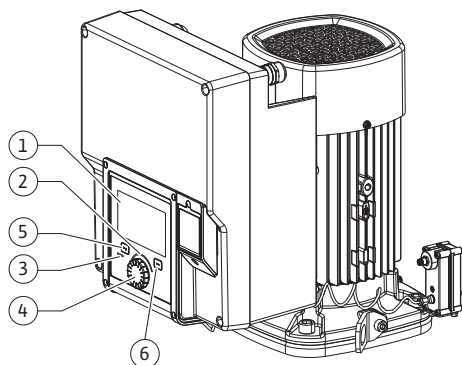
Fig. 33: Ovládací prvky
