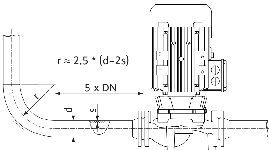
Fig. 13: Uklidňovací úsek před a za čerpadlem
