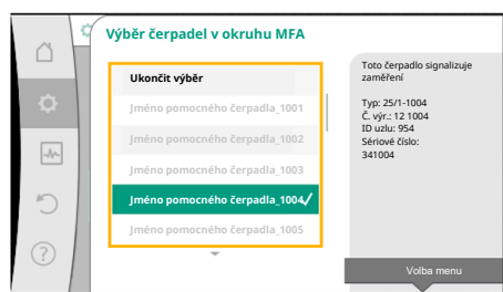
Fig. 63: Výběr sekundárních čerpadel k Multi-Flow Adaptation
