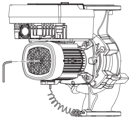
Fig. 5: Otáčení hřídele
