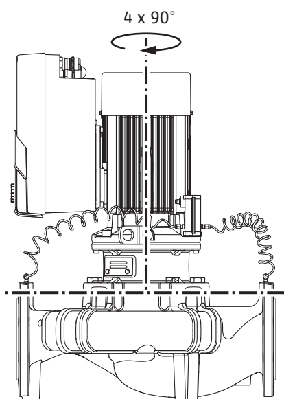
Fig. 11: Přípustné polohy instalace s vertikální hřídelí motoru
