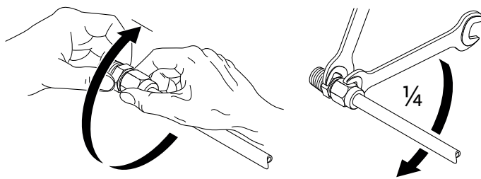
Fig. 14: Otočení šroubů upínacího kroužku o další 1/4 otáčky
