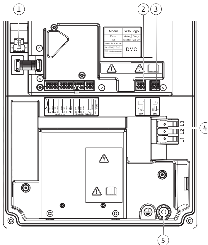
Fig. 24: Přehled svorek v modulu (11 kW ... 22 kW)
