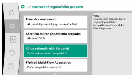
Fig. 62: Průvodce nastavením – volba sekundárních čerpadel
