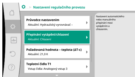
Fig. 52: Přepínání vytápění/chlazení
