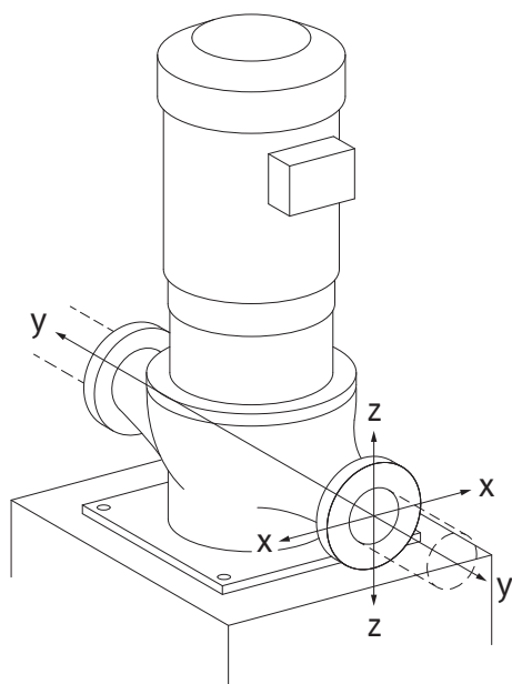
Fig. 16: Příklad zatížení 17A, EN ISO 5199, příloha B
