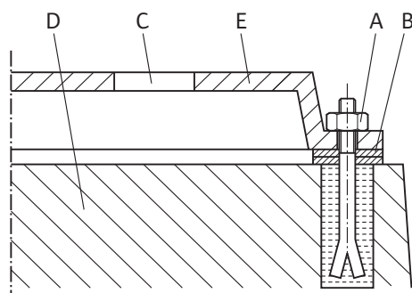
Fig. 10: Příklad pro sešroubování s podkladem
