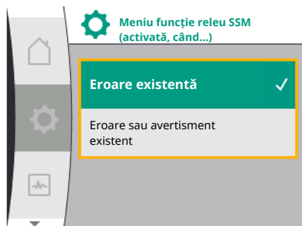
Fig. 60: Meniu funcție releu SSM
