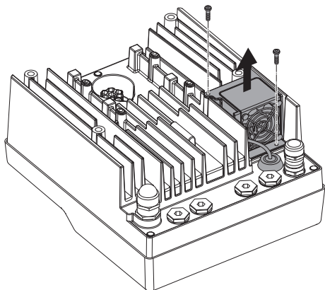
Fig. 108: Demontarea ventilatorului modului
