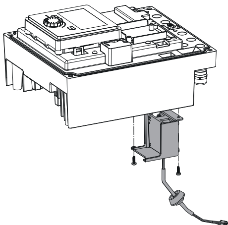
Fig. 109: Scoateți ventilatorul modului, inclusiv cablul și garnitura din cauciuc
