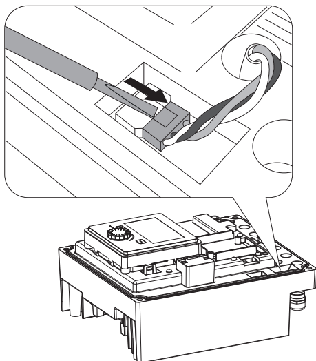
Fig. 107: Deconectarea cablului de conectare al ventilatorului modului
