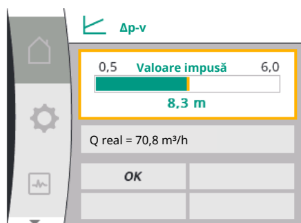
Fig. 32: Reglajul valorii impuse Δp-v ecran de pornire
