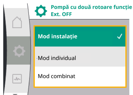
Fig. 68: Moduri selectabile pentru EXT. OFF la pompa cu două rotoare
