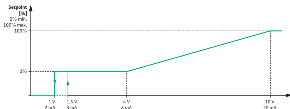
Fig. 79: Comportament semnal analogic AI2: Valoare impusă pentru tipul de semnal 0 ... 10 V/0 ... 20 mA
