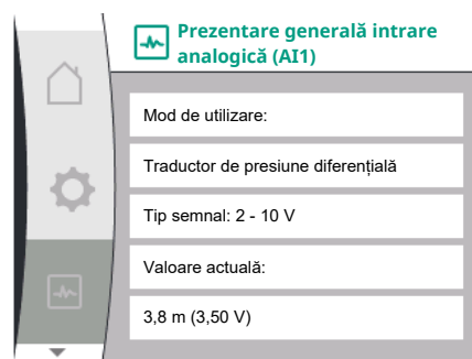
Fig. 96: Prezentare generală intrare analogică (AI1)
