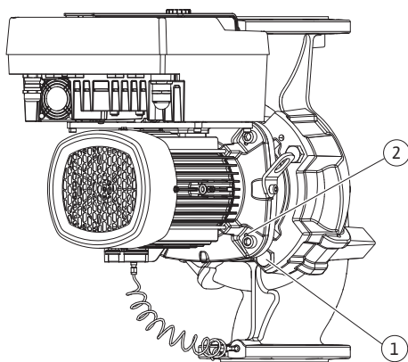
Fig. 105: Apăsarea ansamblului motor cu rotor hidraulic prin găurile filetate (în funcție de tipul pompei)
