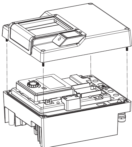
Fig. 106: Deschiderea capacului modului electronic
