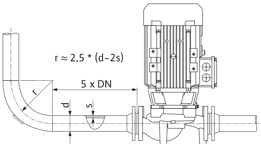
Fig. 12: Stabilizačná trasa pred a za čerpadlom
