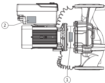
Fig. 2: Typové štítky
