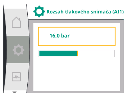
Fig. 71: Nastavenie rozsahu tlakového snímača
