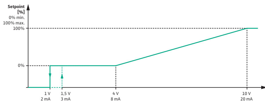
Fig. 79: Správanie analógového signálu AI2: Požadovaná hodnota pri type signálu 0 ... 10 V/ 0 ... 20 mA
