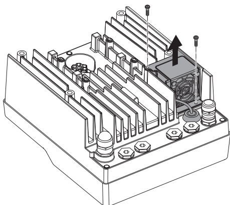
Fig. 108: Demontáž ventilátora modulu
