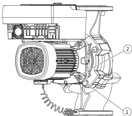
Fig. 105: Odtlačenie nástrčného bloku cez závitové otvory (v závislosti od typu čerpadla)
