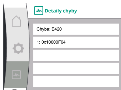
Fig. 93: Menu Detaily chyby
