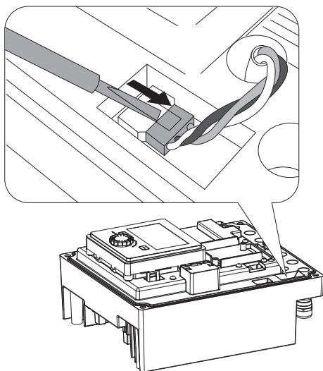
Fig. 107: Uvoľnenie pripojovacieho kábla ventilátora modulu
