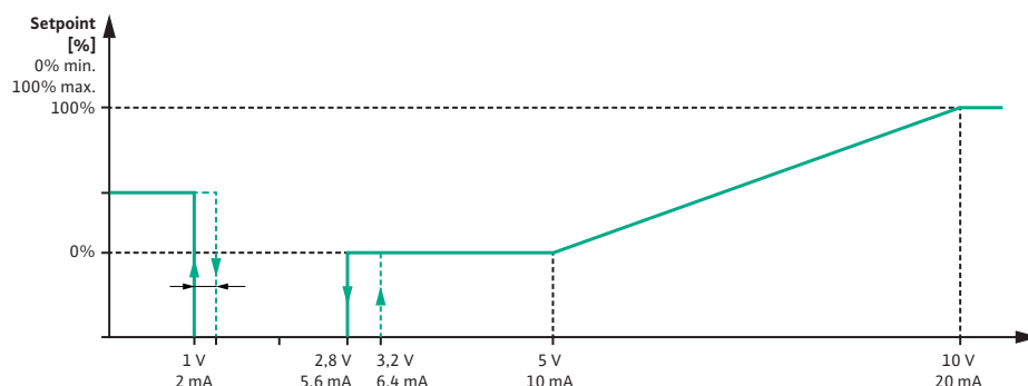
Fig. 78: Comportamento da entrada analógica AI2: Valor nominal com tipo de sinal 2 ... 10 V / 4 ... 20 mA
