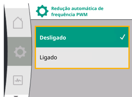
Fig. 87: Menu Redução de frequência PWM
