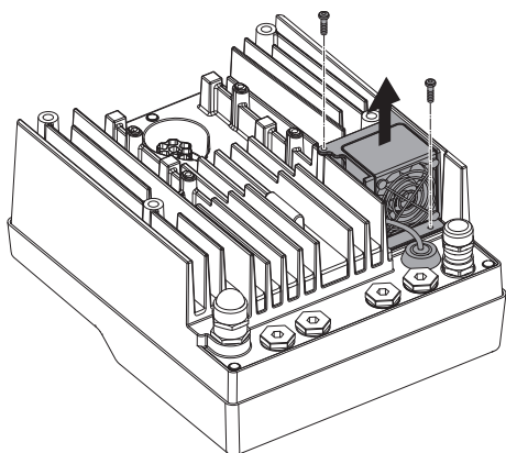
Fig. 108: Desmontagem do ventilador do módulo
