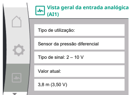
Fig. 96: Vista geral da entrada analógica (AI1)
