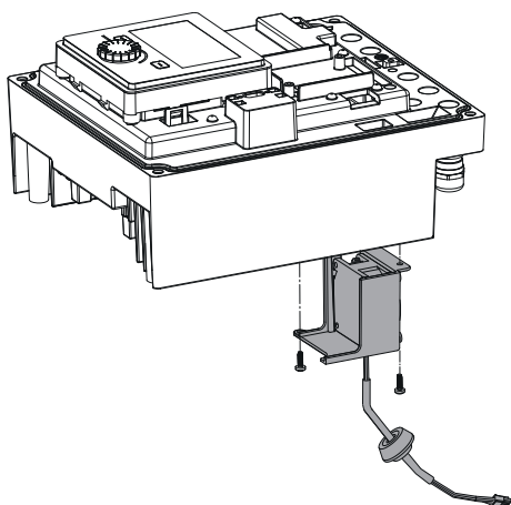
Fig. 109: Retirar o ventilador do módulo, incluindo o cabo e o vedante de borracha
