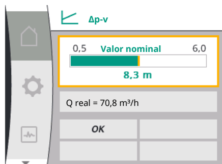
Fig. 32: Ajuste do valor nominal do visor inicial Δp-v
