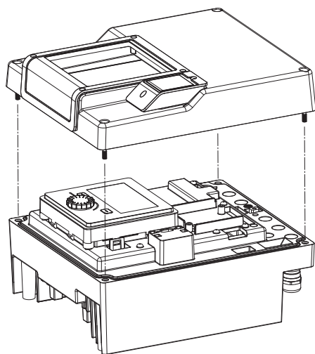
Fig. 106: Abrir a tampa do módulo eletrónico
