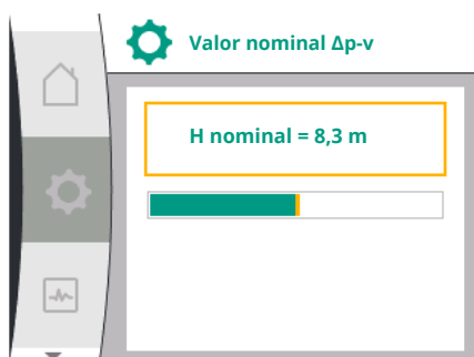
Fig. 40: Regulação do valor nominal Δp-v
