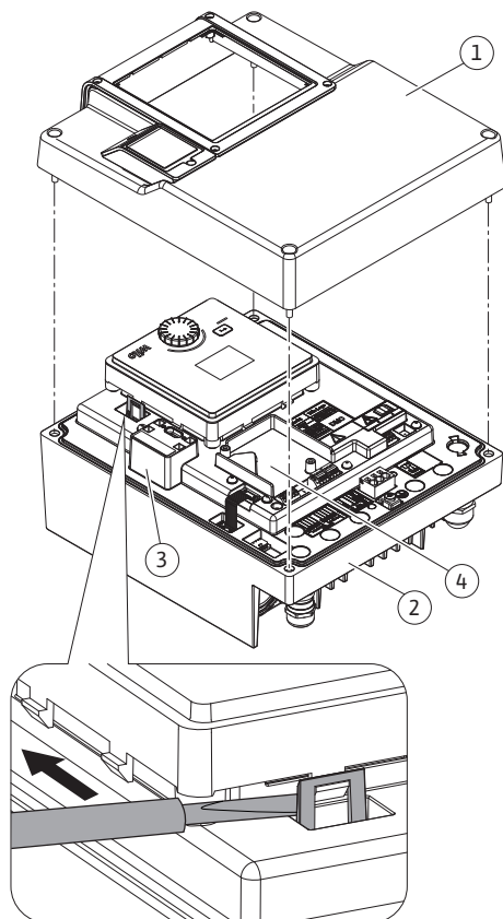
Fig. 26: Módulo eletrónico
