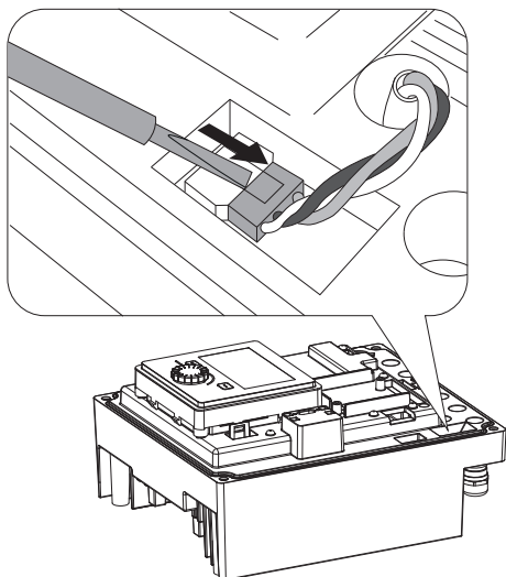
Fig. 107: Desapertar o cabo de ligação do ventilador do módulo
