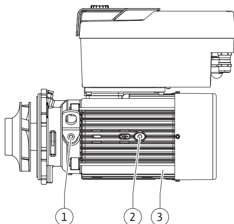
Fig. 4: Unidade de impulsor motor
