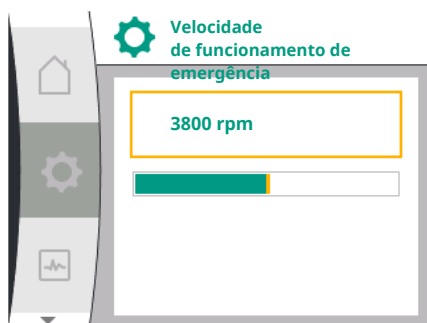
Fig. 45: Velocidade de funcionamento de emergência
