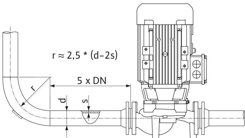
Fig. 12: Izlīdzināšanas posms pirms un pēc sūkņa
