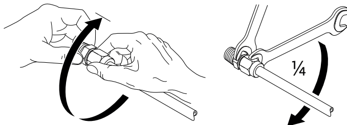
Fig. 13: Turpmāka savilcējgredzena skrūšsavienojuma pagriešana par 1/4 pagriezienu
