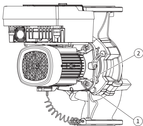
Fig. 105: Ievietojamā moduļa nospiešana, izmantojot vītnes urbumus (atkarībā no sūkņa tipa)
