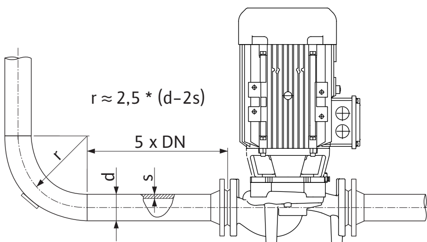
Fig. 12: Percorso di stabilizzazione a monte e a valle della pompa
