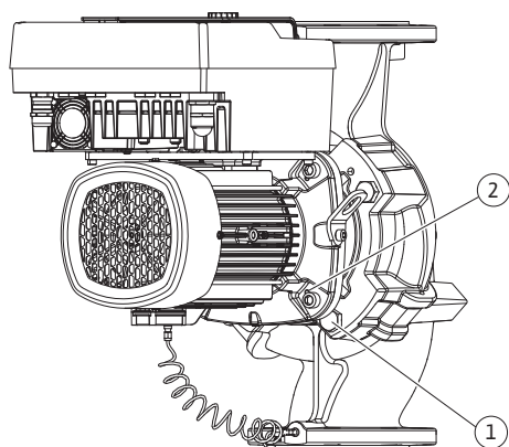
Fig. 105: Estrazione del set di innesto tramite fori filettati (a seconda del tipo di pompa)
