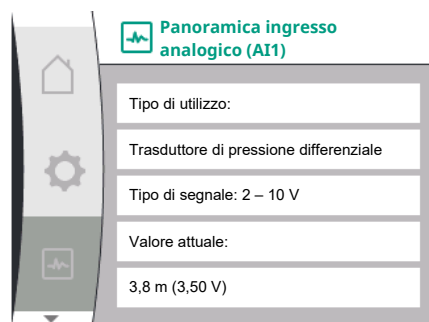
Fig. 96: Panoramica ingresso analogico (AI1)
