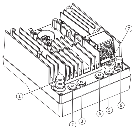
Fig. 19: Pressacavi/passacavi
