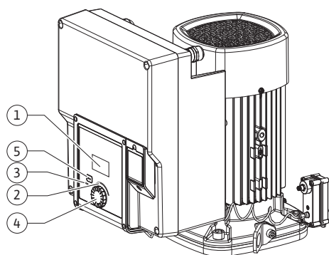
Fig. 27: Elementi di comando
