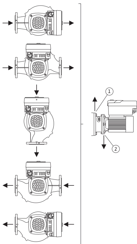
Fig. 9: Posizioni di montaggio ammesse con albero del motore orizzontale
