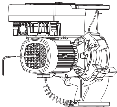
Fig. 5: Rotazione dell'albero
