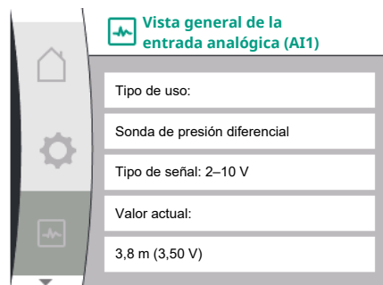
Fig. 96: Vista general de la entrada analógica (AI1)
