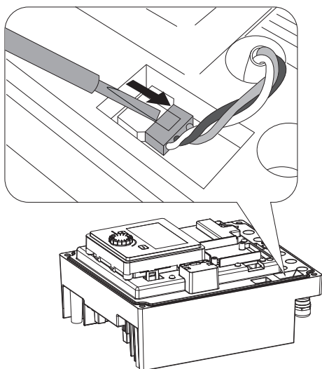
Fig. 107: Soltar el cable de conexión del ventilador del módulo
