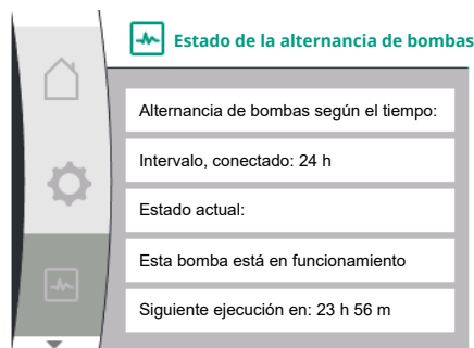
Fig. 98: Información sobre el estado de la alternancia entre las bombas
