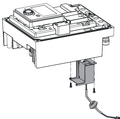
Fig. 109: Retirar el ventilador del módulo, incl. el cable y la junta de goma
