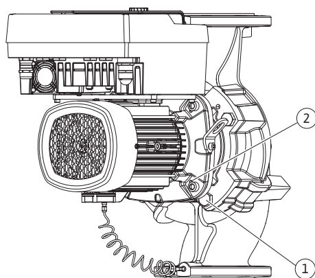
Fig. 105: Expulsión del juego de introducción mediante los taladros roscados (según el modelo de bomba)
