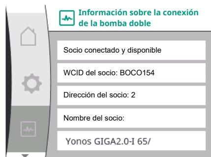
Fig. 97: Información sobre la conexión de bomba doble
