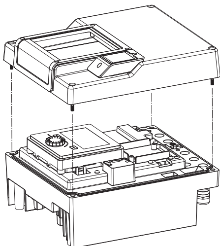
Fig. 106: Abrir la tapa del módulo electrónico
