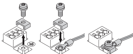
Fig. 22: Εύκαμπτο καλώδιο σύνδεσης
