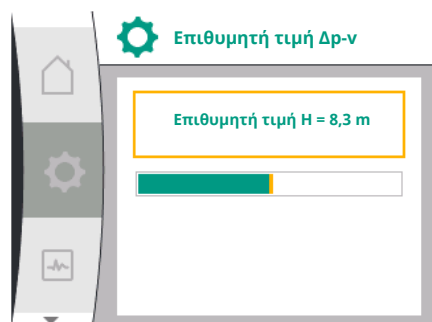
Fig. 40: Ρύθμιση επιθυμητής τιμής Δp-v
