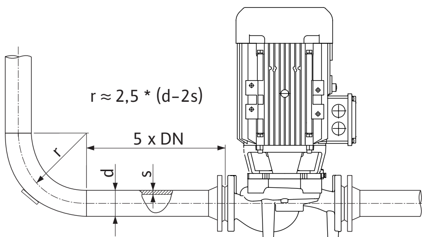
Fig. 12: Διαδρομή ηρεμίας πριν και μετά την αντλία
