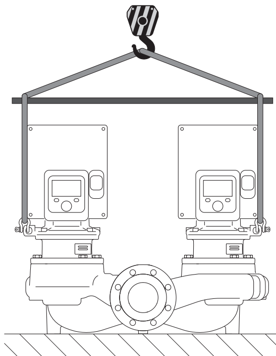
Fig. 7: Διάταξη ανάληψης φορτίου διδυμης αντλίας
