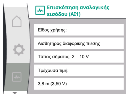
Fig. 96: Επισκόπηση αναλογικής εισόδου (AI1)
