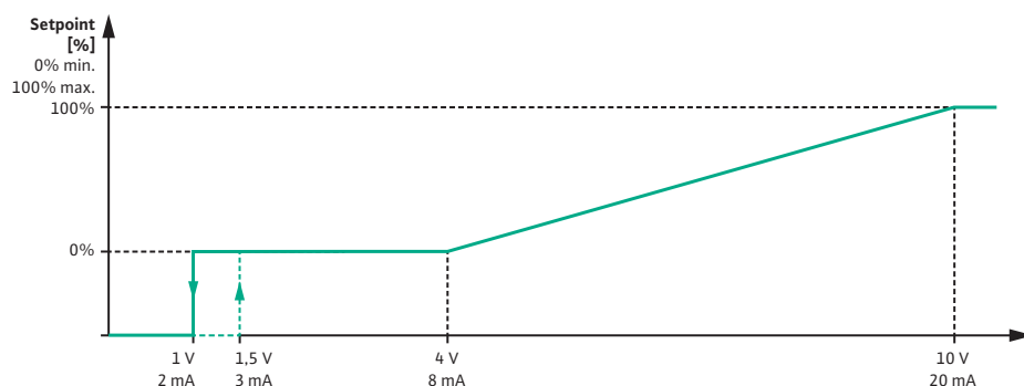
Fig. 79: Συμπεριφορά αναλογικού σήματος AI2: Επιθυμητή τιμή σε τύπο σήματος 0 ... 10 V / 0 ... 20 mA
