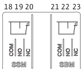
Fig. 24: Ακροδέκτες για SSM και SBM
