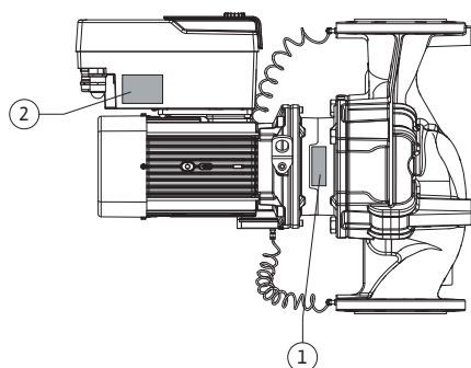
Fig. 2: Πινακίδες στοιχείων προϊόντος
