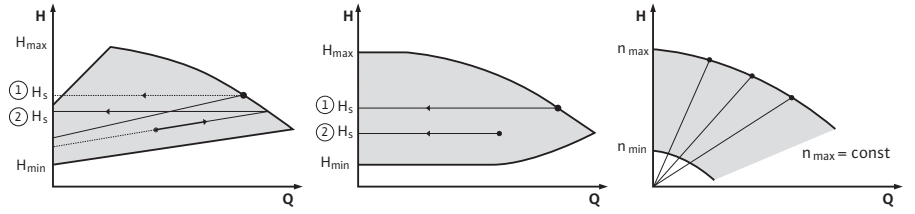
Fig. 38: Regülasyon işlevleri
