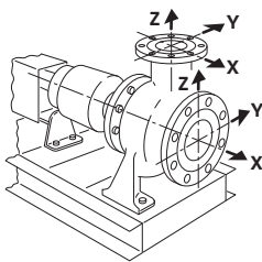
Fig. 15: Yük durumu 1A
