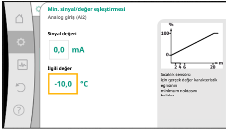
Fig. 87: Min. sinyal/değer eşleştirme gerçek değer sensörü
