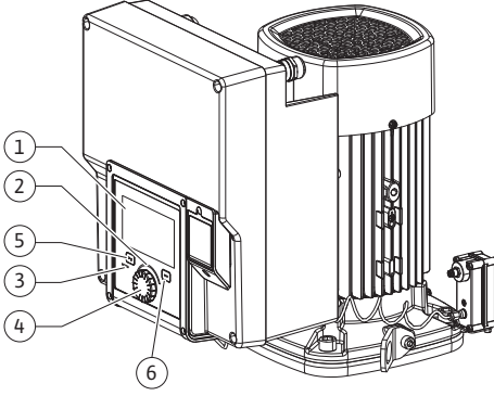
Fig. 29: Kumanda elemanları
