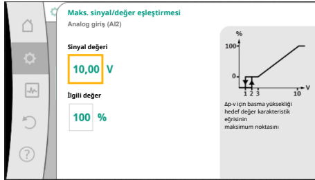
Fig. 83: Maks. sinyal/değer eşleştirme
