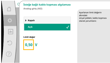
Fig. 79: Limit değeri kablo kopması
