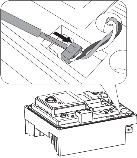
Fig. 110: Modül fanının bağlantı kablosunu çözün
