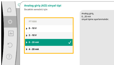
Fig. 86: Sinyal tipi
