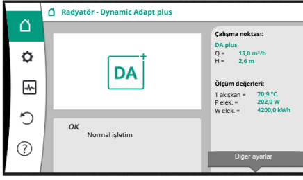
Fig. 33: Ana menü
