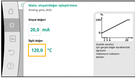
Fig. 88: Maks. sinyal/değer eşleştirme gerçek değer sensörü
