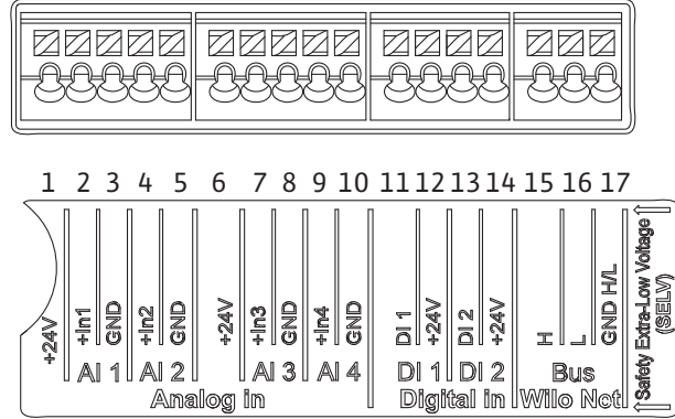
Fig. 21: Analog girişler, dijital girişler ve Wilo Net için klemensler
