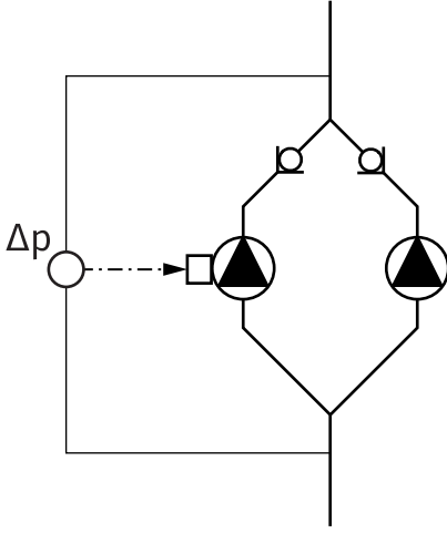
Fig. 18: Örnek – Birleştirme parçası kurulumunda fark basıncı sensörü bağlantısı
