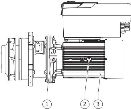
Fig. 4: Takma kiti
