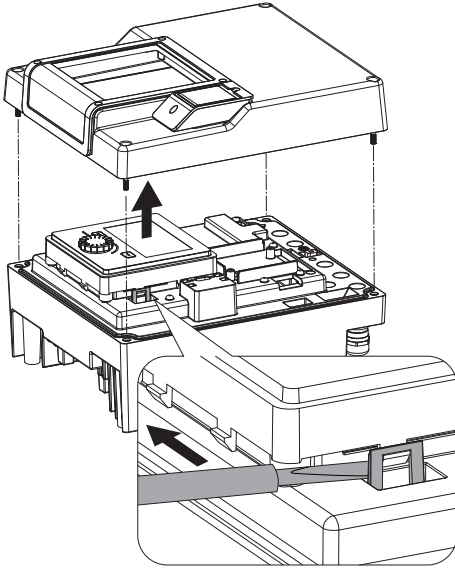
Fig. 113: Modül kapağını söküp; ekranı ve kumanda ünitesini kilitten çıkarın
