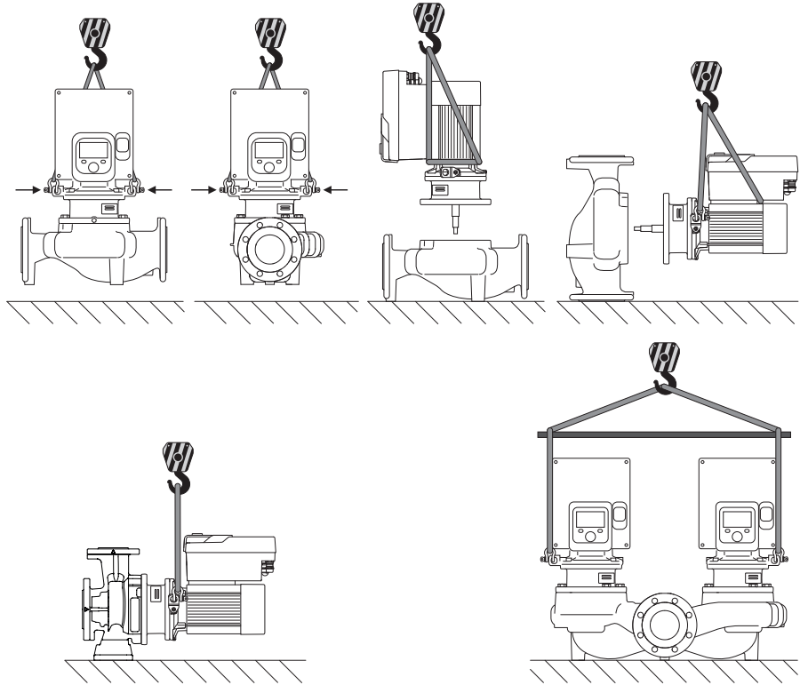
Fig. 6: Kaldırma yönü
