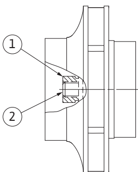
Fig. 107: Pumphjulsmutterns korrekta position efter installationen
