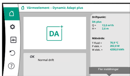
Fig. 33: Huvudmeny
