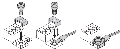
Fig. 22: Flexibel anslutningskabel
