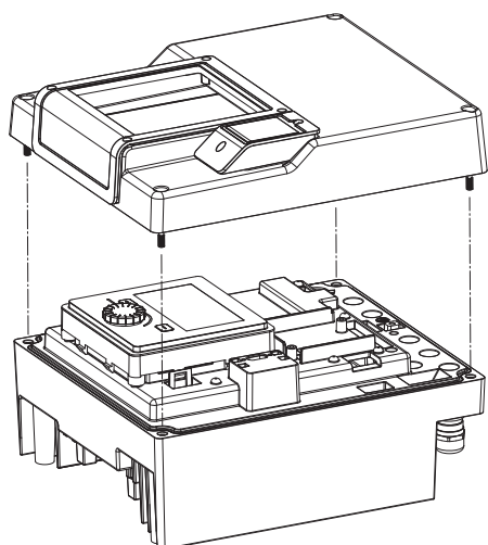
Fig. 109: Öppna elektronikmodulens kåpa
