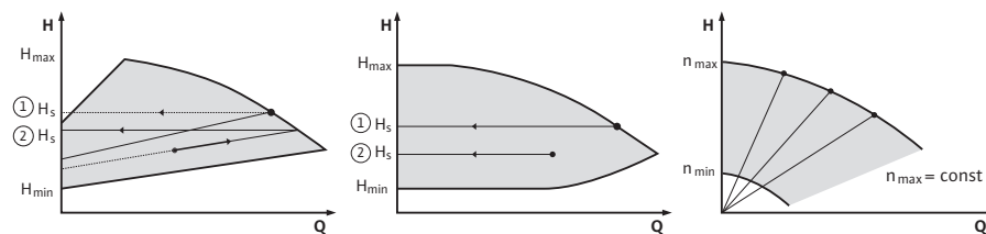
Fig. 38: Regleringsfunktioner
