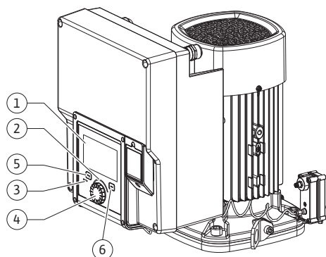
Fig. 29: Manöverelement
