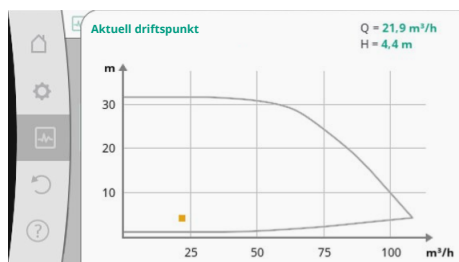
Fig. 96: Aktuell driftspunkt
