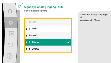
Fig. 86: Signaltyp
