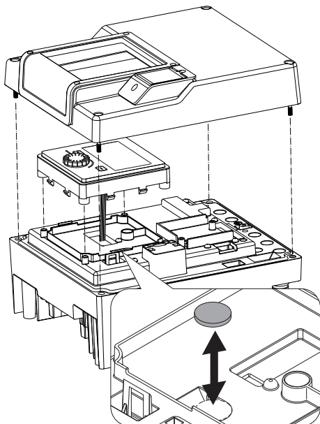
Fig. 114: Lyft display- och manöverenheten och byt ut batteriet
