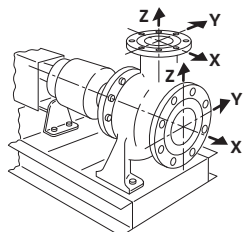
Fig. 15: Lastfall 1A
