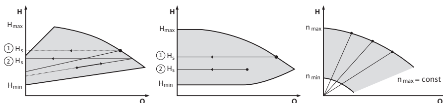
Fig. 38: Funkcije reguliranja
