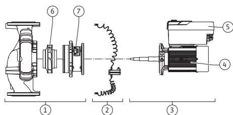
Fig. 3: Funkcijski sklopi
