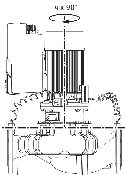
Fig. 9: Dopustni vgradni položaji z navpično gredjo motorja
