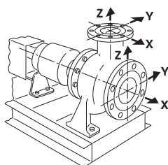
Fig. 15: Zaťažovací stav 1A
