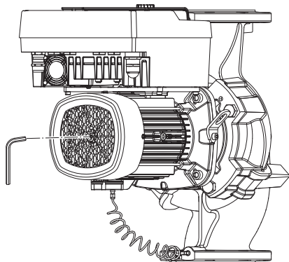
Fig. 5: Točenie hriadeľa
