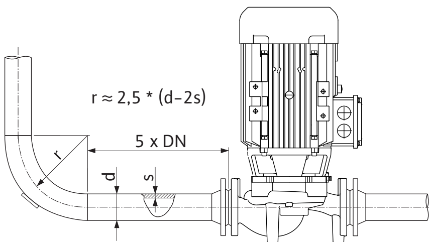
Fig. 11: Stabilizačná trasa pred a za čerpadlom
