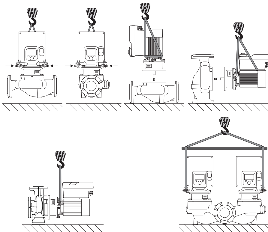
Fig. 6: Zdvíhacie zariadenie
