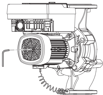
Fig. 5: Вращение вала
