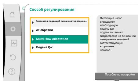
Fig. 56: Пример способа регулирования Multi-Flow Adaptation
