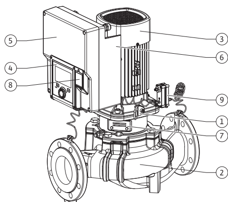
Fig. 1: Обзор насоса
