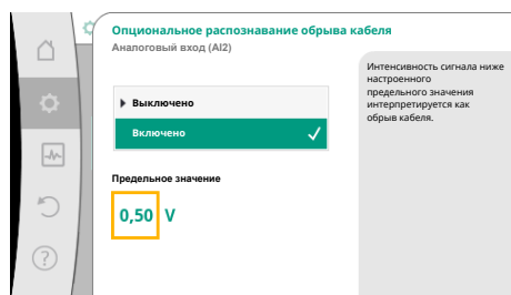
Fig. 79: Предельное значение, обрыв кабеля
