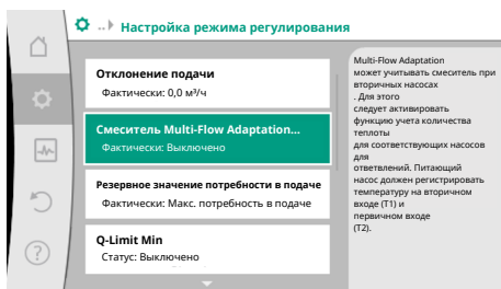
Fig. 60: Настройка режима регулирования: Смеситель Multi-Flow Adaptation
