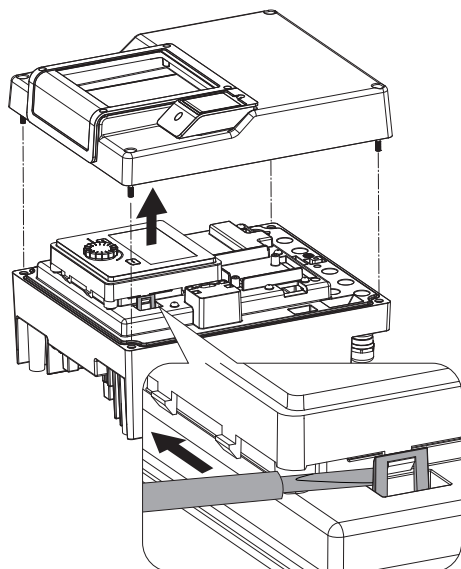
Fig. 113: Demontați capacul modulului; eliberați unitatea de display și operare din elementul de blocare
