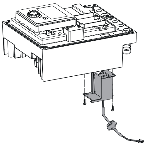
Fig. 112: Scoateți ventilatorul modului, inclusiv cablul și garnitura din cauciuc
