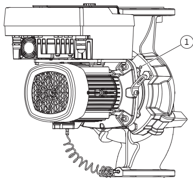
Fig. 104: Apăsarea ansamblului motor cu rotor hidraulic prin găurile filetate
