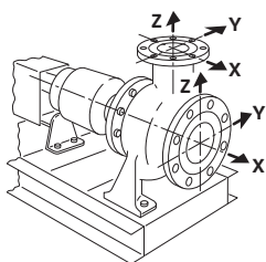
Fig. 15: Caz de încărcare 1A
