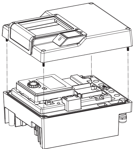
Fig. 109: Abrir a tampa do módulo eletrônico
