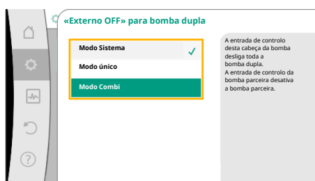
Fig. 66: Modos seleccionáveis para EXT. OFF em bombas duplas
