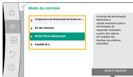
Fig. 56: Exemplo de modo de controlo «Multi-Flow Adaptation»
