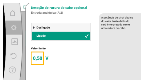
Fig. 79: Valor limite para rutura de cabo
