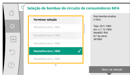
Fig. 59: Seleção das bombas secundárias para Multi-Flow Adaptation
