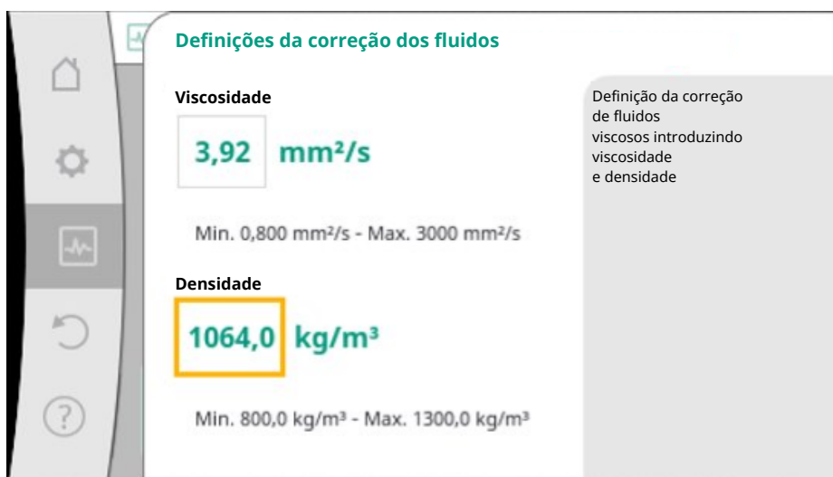
Fig. 98: Regulação da viscosidade e densidade
