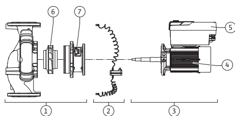
Fig. 3: Módulos funcionais
