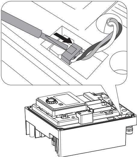
Fig. 110: Løsne tilkoblingskabelen til modulventilatoren
