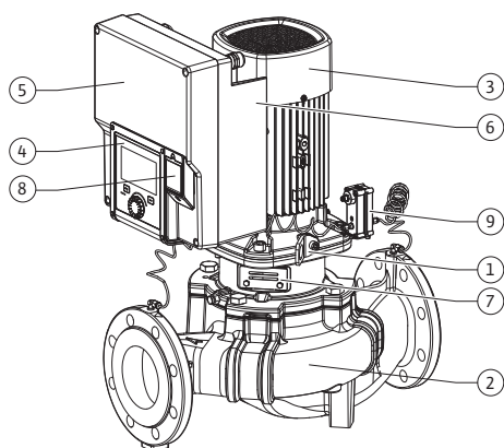
Fig. 1: Oversikt pumpe
