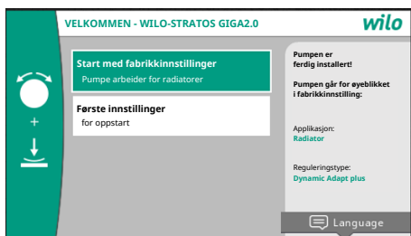
Fig. 32: Meny for førsteinnstillinger
