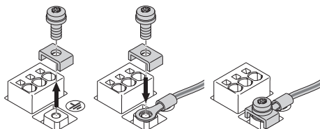
Fig. 22: Fleksibel tilkoblingskabel
