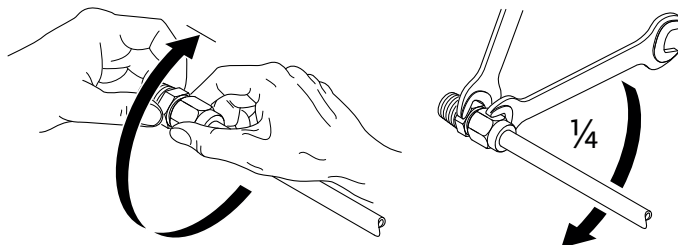
Fig. 12: Dreie klemringskrutilkoblingen 1/4 omdreining til
