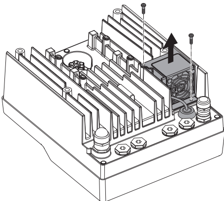
Fig. 111: Demontering av modulventilatoren
