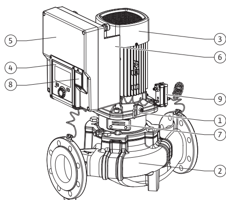
Fig. 1: Overzicht pomp
