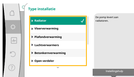
Fig. 42: Voorbeeld installatietype „Radiator”
