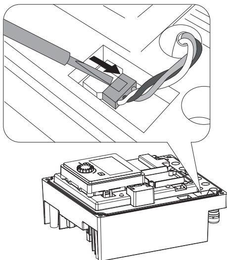
Fig. 110: Moduļa ventilatora pieslēguma kabeļa atvienošana
