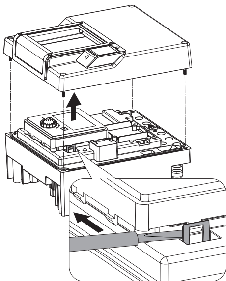
Fig. 113: Moduļa vāka demontāža; displeja un vadības ierīces atbrīvošana no fiksatora
