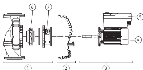
Fig. 3: Funkcionālie mezgli
