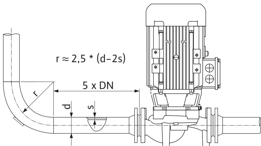
Fig. 11: Izlīdzināšanas posms pirms un pēc sūkņa
