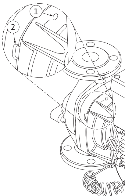
Fig. 105: Vītņu urbumi un atvērumi ievietojamā moduļa izņemšanai no sūkņa korpusa
