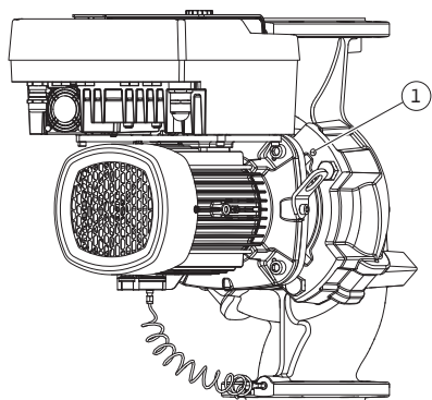
Fig. 104: Ievietojamā moduļa nospiešana, izmantojot vītnes urbumus
