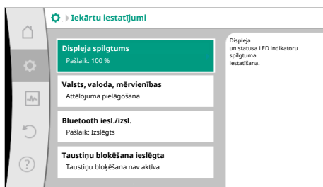
Fig. 91: Iekārtu iestatījumi
