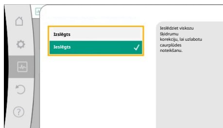
Fig. 97: Šķidrumu korekcija
