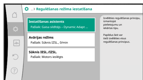
Fig. 44: Iestatīšanas asistents
