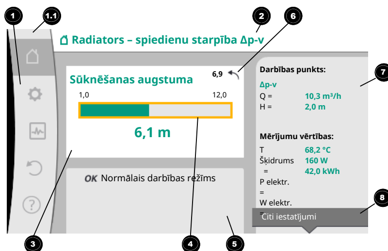
Fig. 34: Sākuma ekrāns
