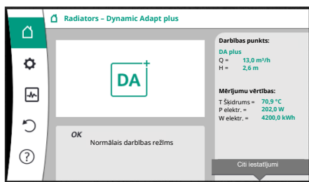
Fig. 33: Galvenā izvēlne
