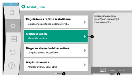
Fig. 35: Iestatījumu izvēlne
