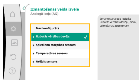
Fig. 36: Iestatījumu dialogs
