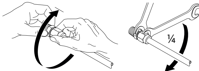
Fig. 12: Turpmāka savilcējgredzena skrūšsavienojuma pagriešana par 1/4 pagriezienu
