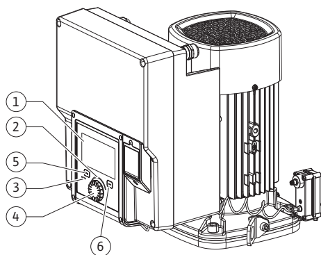
Fig. 29: Vadības elementi
