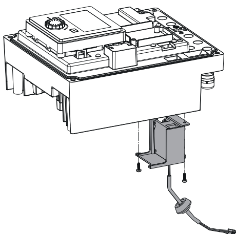
Fig. 112: Moduļa ventilatora, tostarp kabeļa un gumijas blīvējuma, noņemšana
