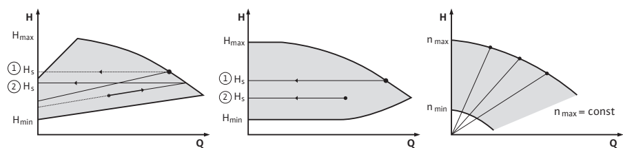
Fig. 38: Regulēšanas funkcijas
