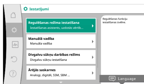
Fig. 39: Iestatīšanas izvēlne
