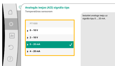
Fig. 86: Signāla veids
