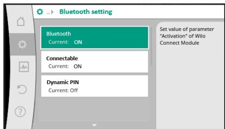
Fig. 90: Bluetooth saskarne
