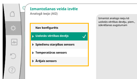
Fig. 75: Iestatījumu dialogs
