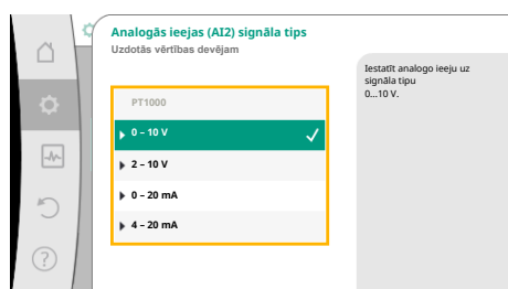
Fig. 76: Signāla veids
