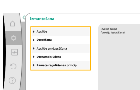
Fig. 40: Pielietojuma izvēle
