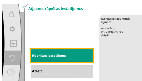
Fig. 101: Rūpnīcas iestatījums
