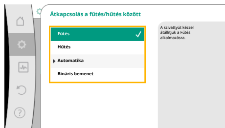
Fig. 49: Átkapcsolás a fűtés/hűtés között_Fűtés
