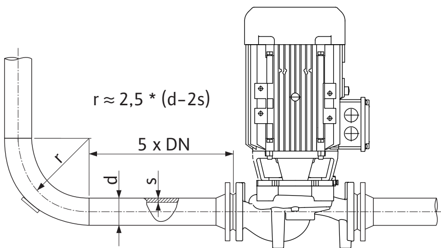
Fig. 11: A szivattyú előtti és utáni csillapítási szakasz
