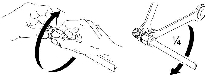
Fig. 12: A szorítógyűrű-csavarokötés 1/4-fordulattal történő továbbforgatása
