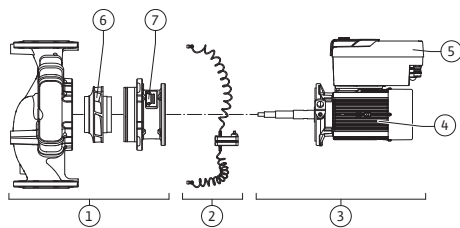
Fig. 3: Funkcionális részegységek
