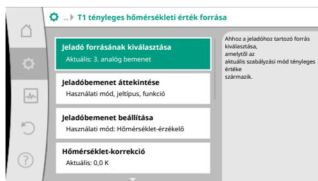
Fig. 63: T1 tényleges hőmérsékleti érték forrása
