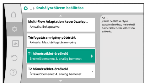
Fig. 62: Multi-Flow Adaptation keverőselelep: Hőmérséklet-érzékelő
