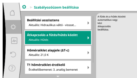
Fig. 48: Átkapcsolás a fűtés/hűtés között
