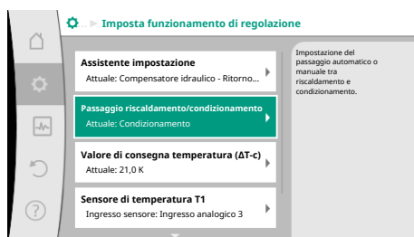
Fig. 48: Passaggio riscaldamento/condizionamento
