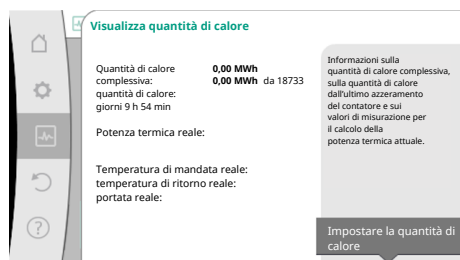
Fig. 94: Visualizza quantità di calore
