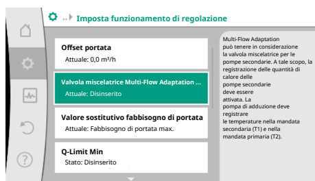
Fig. 60: Imposta funzionamento di regolazione: Valvola miscelatrice Multi-Flow Adaptation
