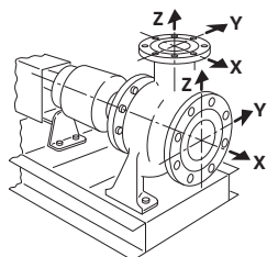
Fig. 15: Tipologia di carico 1A
