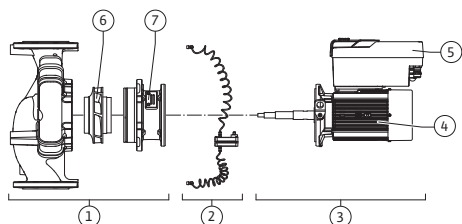
Fig. 3: Moduli funzionali
