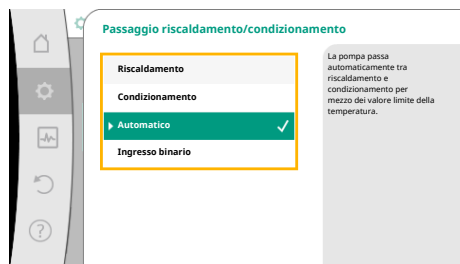
Fig. 51: Passaggio riscaldamento/condizionamento_Automatico
