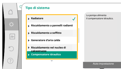
Fig. 55: Tipo di sistema “Compensatore idraulico”
