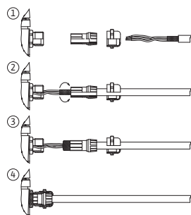
Fig. 25: Supporto schermato
