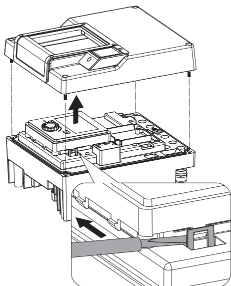
Fig. 113: Demontaža poklopca modula; otpuštanje zaslona i kontrolne jedinice iz zapora
