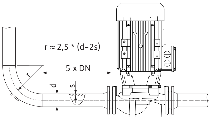
Fig. 11: Stabilizacijska dionica ispred i iza pumpe
