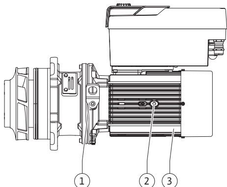
Fig. 4: Utični komplet
