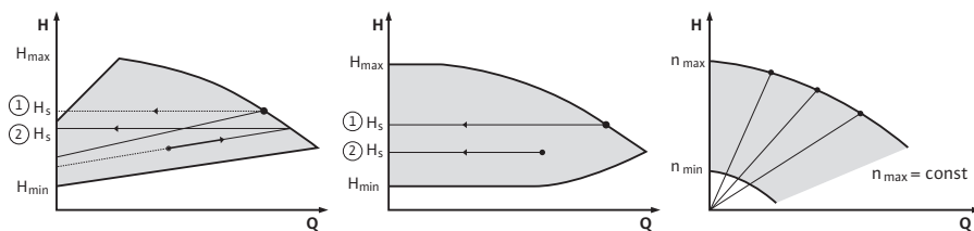
Fig. 38: Funkcije regulacije
