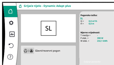
Fig. 65: Početni zaslon partnera dvostruke pumpe bez montiranog senzora diferencijalnog tlaka
