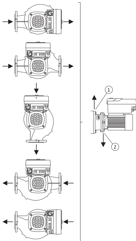
Fig. 17: Dopusćeni položaji ugradnje s vodoravnim vratilom
