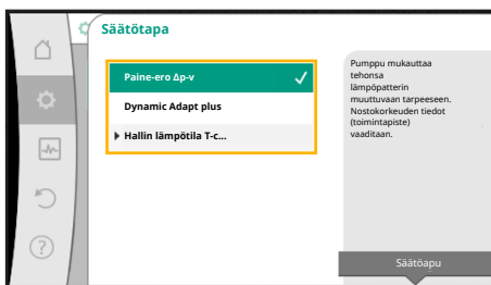
Fig. 31: Keltainen keskiö: Asetusten muutokset
