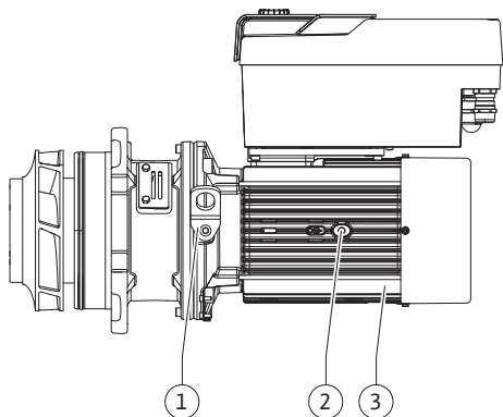
Fig. 4: Moottori-juoksupyöräyksikkö
