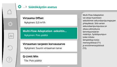
Fig. 60: Säätökäytön asetus: Multi-Flow Adaptation –sekoitin
