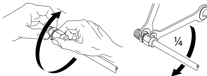
Fig. 12: Kiristysrengasruuviiliitoksen kääntäminen edelleen 1/4-kierrosta
