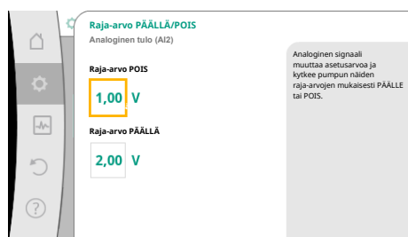
Fig. 81: Raja-arvot PÄÄLLE-/POIS-ohjaukseen analogisten signaalien kautta
