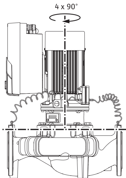
Fig. 9: Sallitut asennusasennot, pystysuuntainen moottoriakseli
