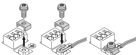
Fig. 23: Cable de conexión rígido
