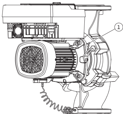
Fig. 104: Expulsión del juego de introducción mediante los taladros roscados
