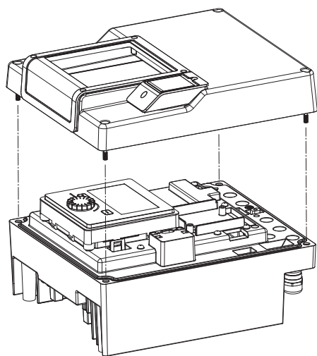
Fig. 109: Abrir la tapa del módulo electrónico
