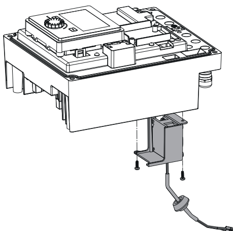
Fig. 112: Retirar el ventilador del módulo, incl. el cable y la junta de goma
