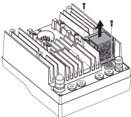
Fig. 111: Desmontaje del ventilador del módulo
