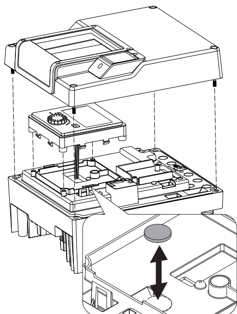
Fig. 114: Elevar la unidad de pantalla y control, sustituir la batería
