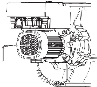
Fig. 5: Giro del eje
