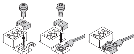
Fig. 22: Cable de conexión flexible
