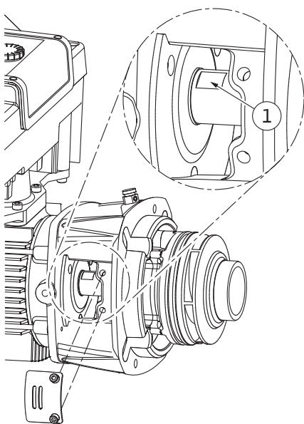
Fig. 106: Planos de llave en el eje
