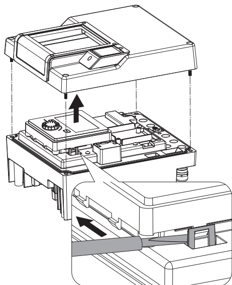
Fig. 113: Desmontar la tapa del módulo; soltar la unidad de pantalla y control del dispositivo de bloqueo
