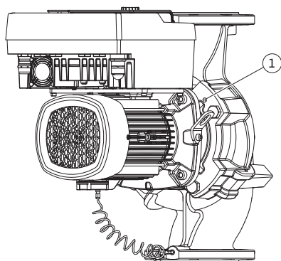
Fig. 10: Expulsión del juego de introducción mediante los taladros roscados
