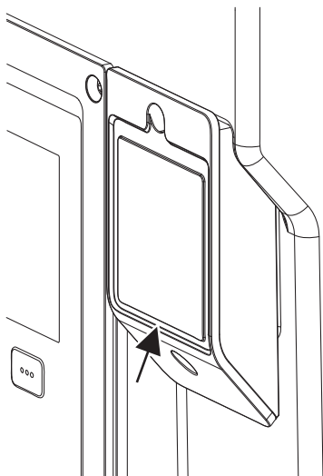
Fig. 28: Tapa para el módulo Wilo-Smart Connect BT
