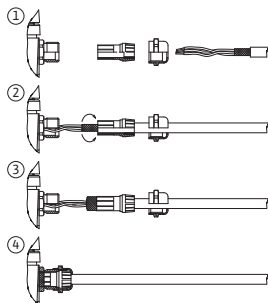
Fig. 25: Schirmauflage
