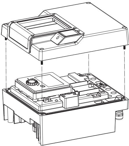
Fig. 109: Deckel des Elektronikmoduls öffnen
