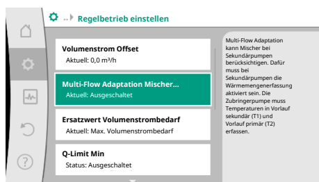
Fig. 60: Regelbetrieb einstellen: Multi-Flow Adaptation Mischer
