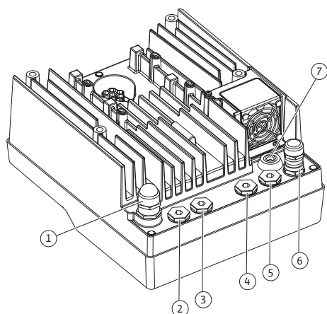
Fig. 19: Kabelverschraubungen/Kabeldurchführungen
