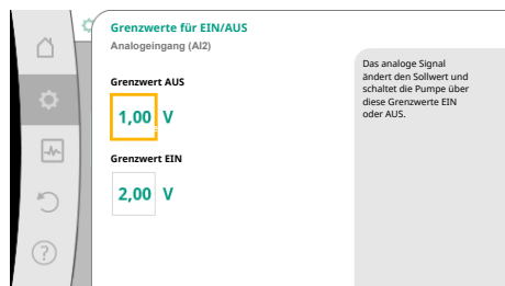
Fig. 81: Grenzwerte zur EIN/AUS-Steuerung über Analogsignale
