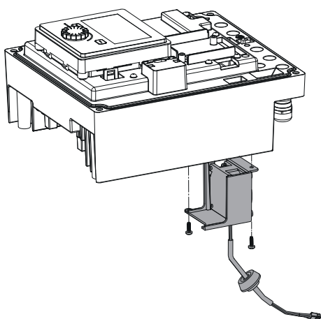
Fig. 112: Modüllüfter inkl. Kabel und Gummidichtung abnehmen
