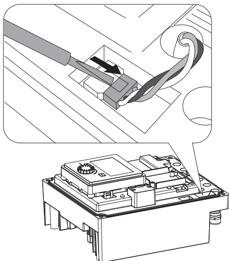
Fig. 110: Uvolnit přírodní kabel ventilátoru modulu
