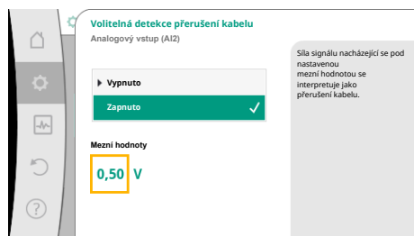
Fig. 79: Mezní hodnota – přerušení kabelu
