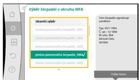
Fig. 59: Výběr sekundárních čerpadel k Multi-Flow Adaptation
