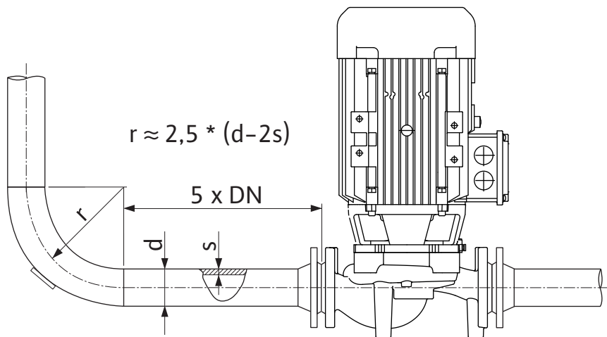
Fig. 11: Uklidňovací úsek před a za čerpadlem
