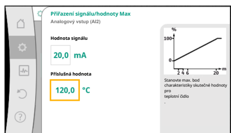
Fig. 88: Přifazení signálu/hodnoty max – ukazatel skutečné hodnoty
