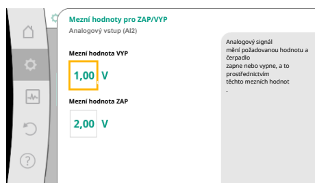
Fig. 81: Mezní hodnoty pro řízení zap/vyp prostřednictvím analogových signálů
