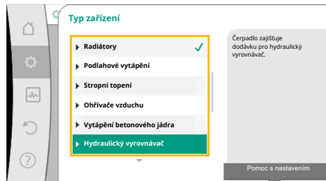
Fig. 55: Typ zařízení „Hydraulický vyrovnávač“
