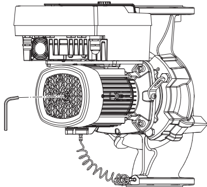
Fig. 5: Otáčení hřídele
