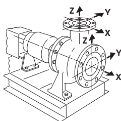
Fig. 15: Příklad zatížení 1A
