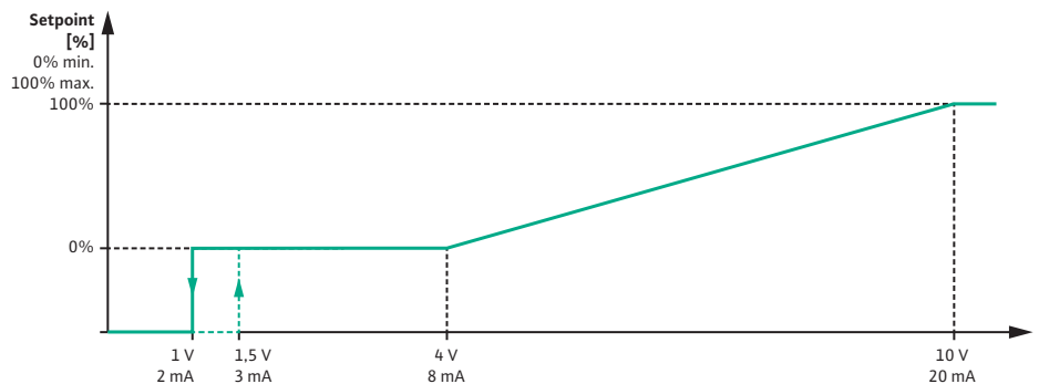
Fig. 79: Поведінка аналогового сигналу AI2: задане значення при типі сигналу 0 – 10 V/0 – 20 mA
