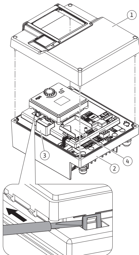
Fig. 26: Електронний модуль
