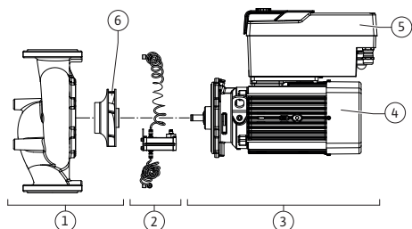
Fig. 3: Функціональні вузли
