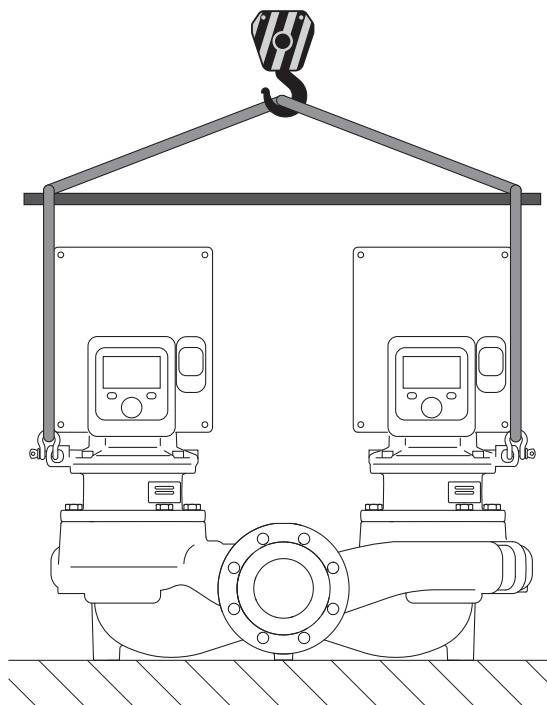
Fig. 7: Напрямок підймання здвоєного насоса
