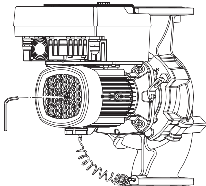
Fig. 5: Повертання вала
