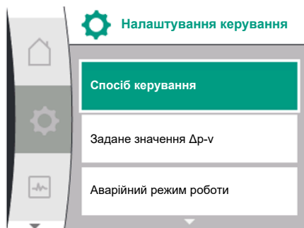
Fig. 38: Спосіб керування
