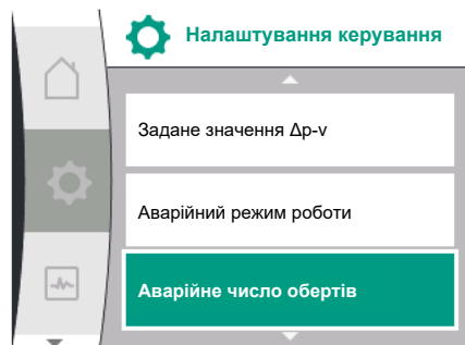
Fig. 73: Меню налаштування керування з режимом аварійної роботи при несправності значення давача
