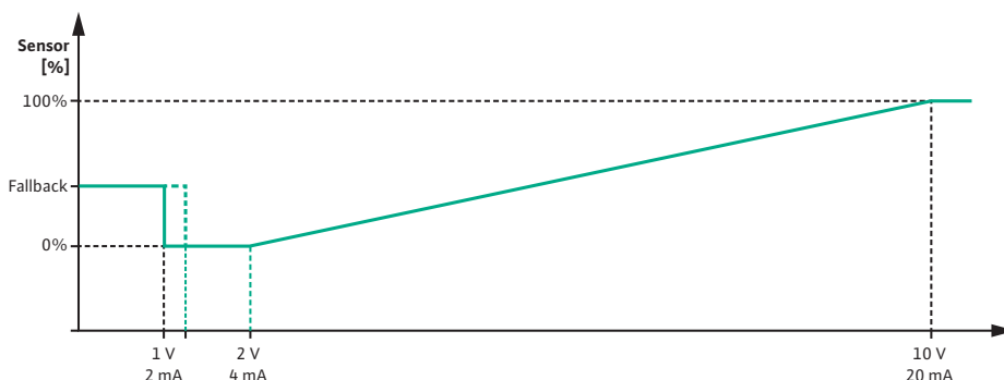
Fig. 72: Поведінка аналогового входу AI 1: значення давача при типі сигналу 2 – 10 V/4 – 20
