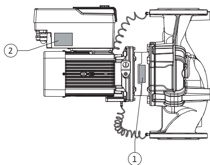
Fig. 2: Заводські таблички
