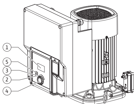
Fig. 27: Bedieningselementen
