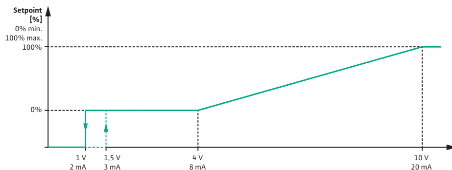
Fig. 79: Gedrag analog signaal AI2: Gewenste waarde bij signaaltipe 0...10 V / 0...20 mA
