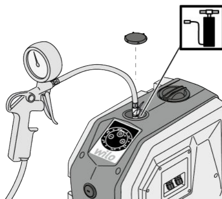
Fig. 12: Naplnenie membránovej expanznej nádoby
