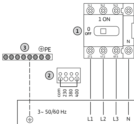
Fig. 3: Alimentazione di rete Control EC-rh
