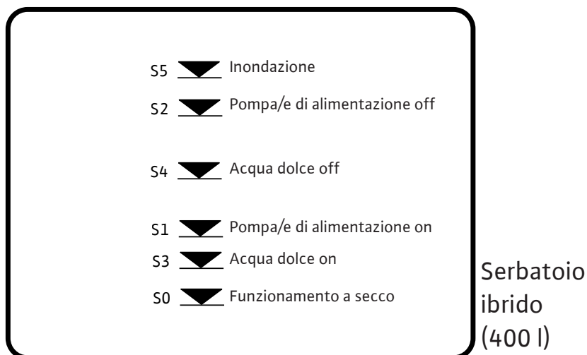
Fig. 20: Funzionamento con trasmettitore di livello
