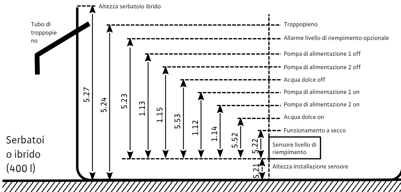
Fig. 19: Parametri di impostazione del serbatoio ibrido
