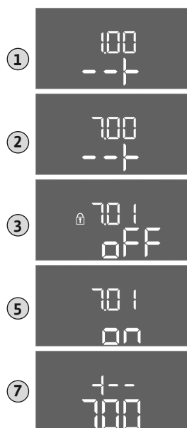
Fig. 22: Abilitazione dell'immissione di parametri
