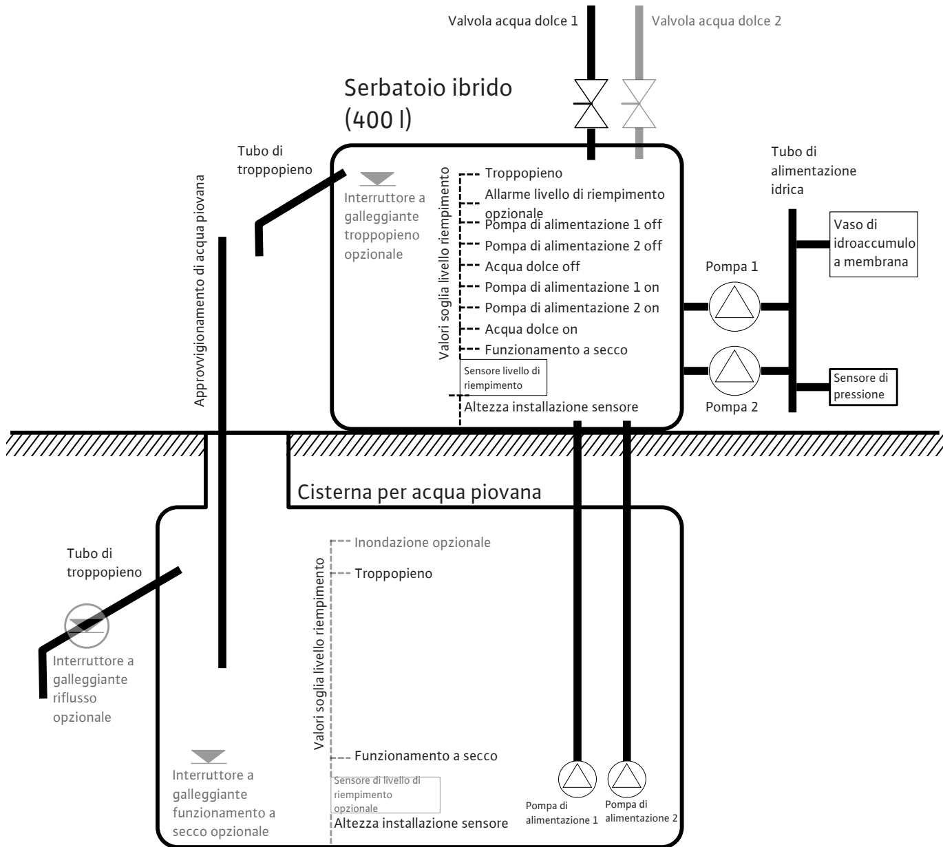
Fig. 17: Principio di funzionamento di AF400 con sensore di livello nel serbatoio ibrido e nella cisterna
