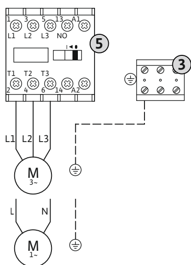
Fig. 4: Raccordement de la pompe
