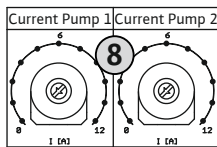
Fig. 5: Réglage du courant nominal du moteur sur le potentiomètre
