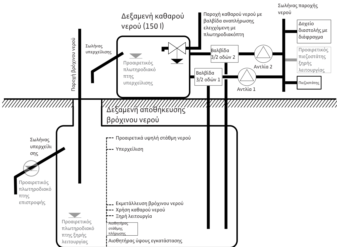
Fig. 20: Σχηματική απεικόνιση της αρχής λειτουργίας του συστήματος AF150
