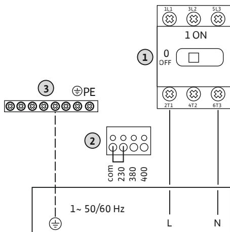
Fig. 3: Ηλεκτρική σύνδεση Control EC-rF
