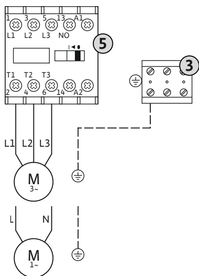
Fig. 4: Σύνδεση αντλίας
