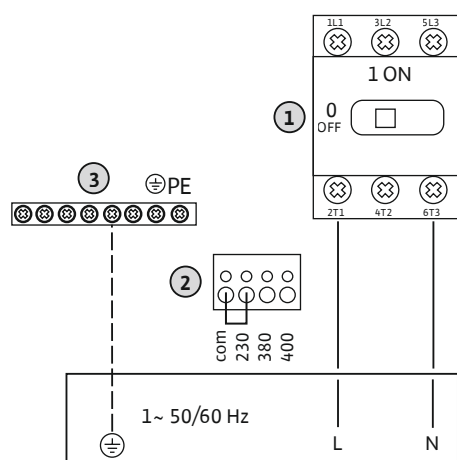
Fig. 3: Síťová přípojka Control EC-rF
