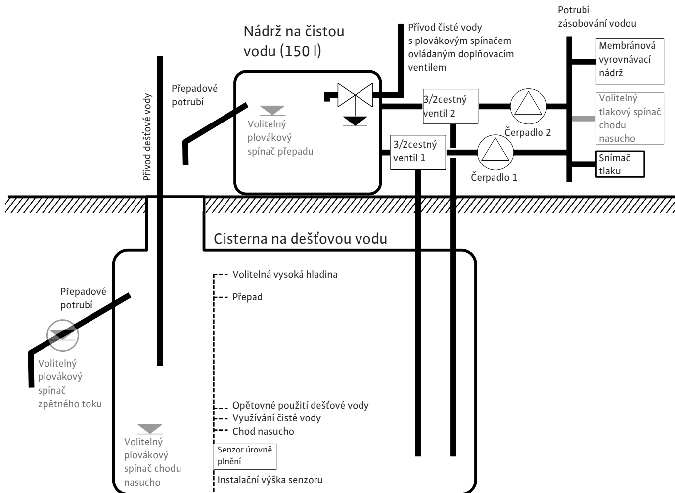
Fig. 20: Schematicky znázorněný princip funkce AF150
