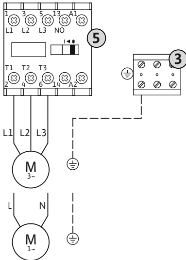
Fig. 6: 水泵接口
